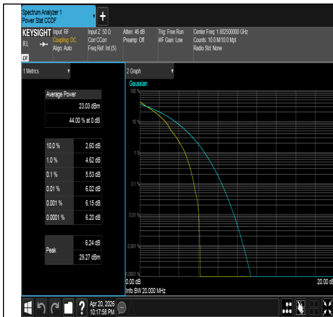
Band25-20MHz-QPSK-26365-1RB#0-PASS
