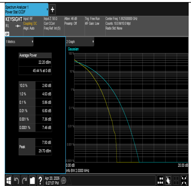
Band25-1.4MHz-QPSK-26365-6RB#0-PASS
