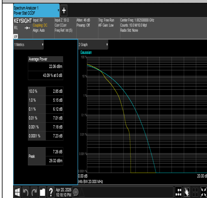
Band25-20MHz-16QAM-26365-1RB#0-PASS
