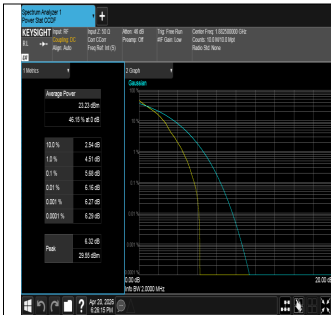
Band25-1.4MHz-QPSK-26365-1RB#0-PASS
