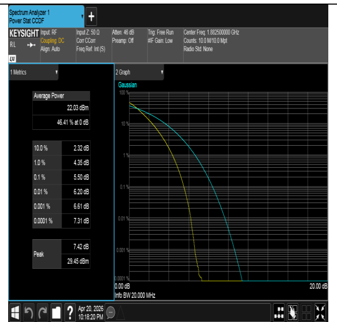
Band25-20MHz-QPSK-26365-100RB#0-PASS
