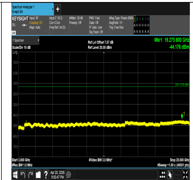
Band25-20MHz-QPSK-26365-1RB#99-3000~20000-PASS
