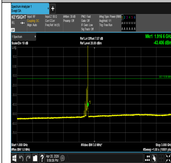
Band25-20MHz-QPSK-26590-1RB#99-1000~3000-PASS
