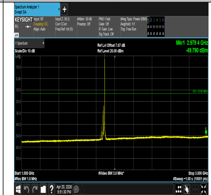
Band25-20MHz-16QAM-26365-1RB#99-1000~3000-PASS
