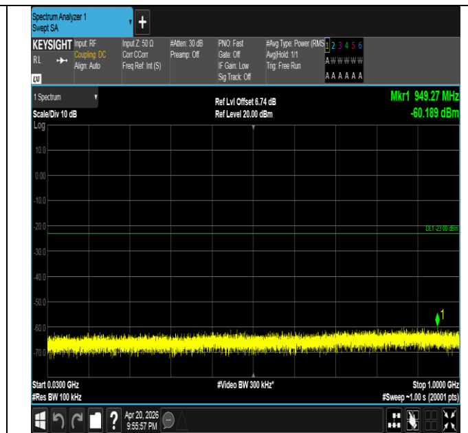
Band25-20MHz-QPSK-26590-1RB#99-30~1000-PASS
