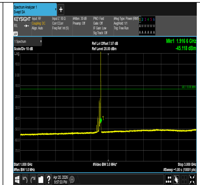
Band25-20MHz-16QAM-26590-1RB#99-1000~3000-PASS
