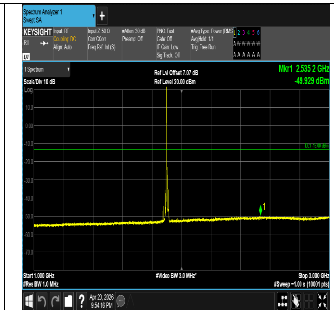
Band25-20MHz-QPSK-26590-1RB#0-1000~3000-PASS
