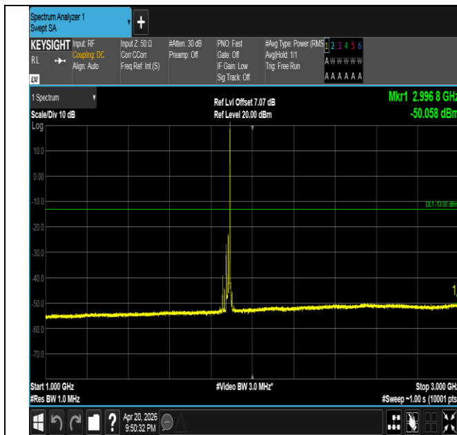
Band25-20MHz-QPSK-26365-1RB#99-1000~3000-PASS
