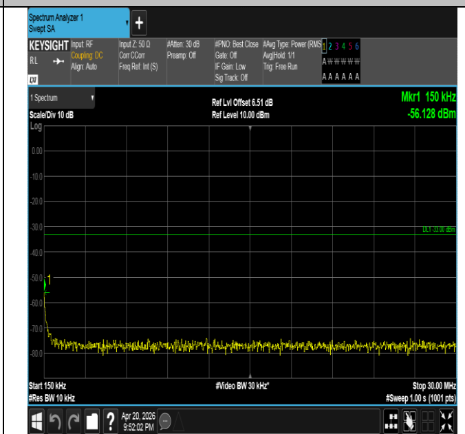
Band25-20MHz-QPSK-26365-100RB#0-0.15~30-PASS
