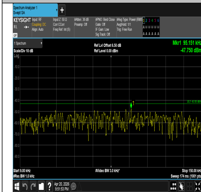
Band25-20MHz-QPSK-26365-100RB#0-0.009~0.15-PASS
