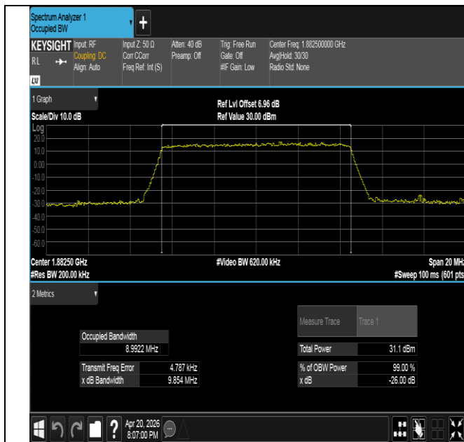
Band25-10MHz-QPSK-26365-50RB#0-PASS
