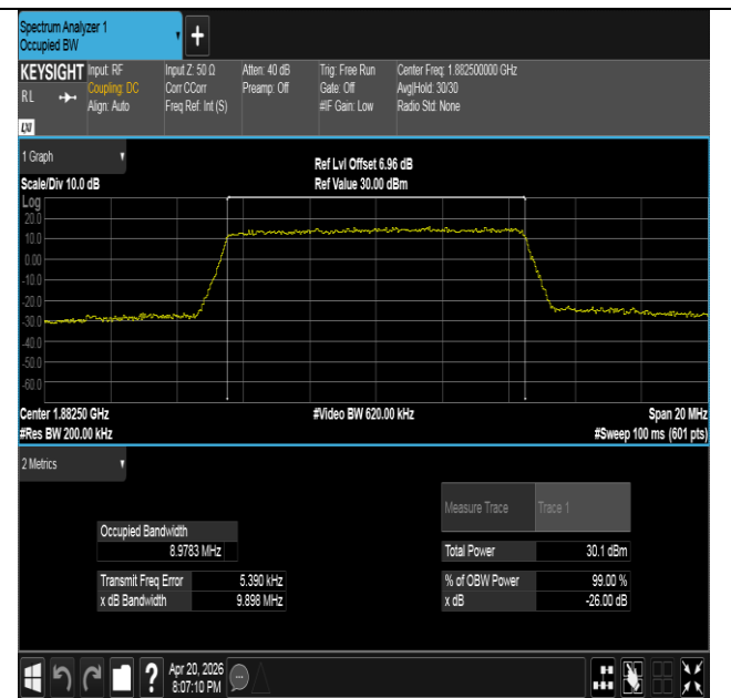
Band25-10MHz-16QAM-26365-50RB#0-PASS
