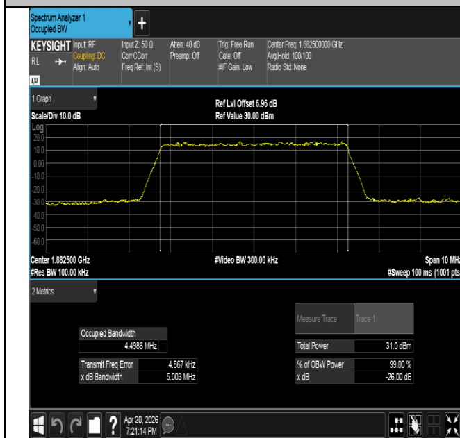
Band25-5MHz-QPSK-26365-25RB#0-PASS
