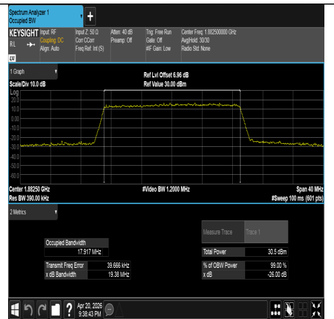
Band25-20MHz-16QAM-26365-100RB#0-PASS
