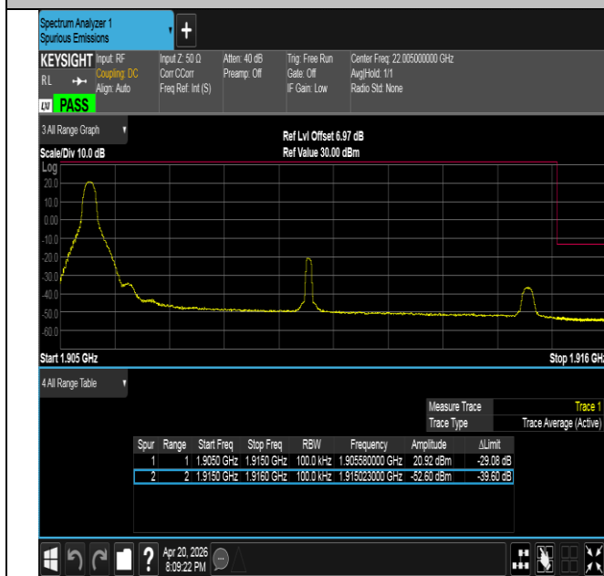
Band25-10MHz-QPSK-26640-1RB#0-PASS
