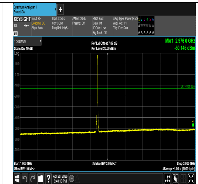
Band25-3MHz-QPSK-26365-15RB#0-1000~3000-PASS
