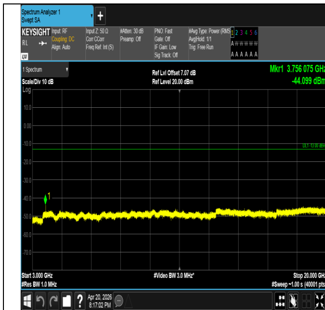
Band25-10MHz-QPSK-26365-1RB#0-3000~20000-PASS
