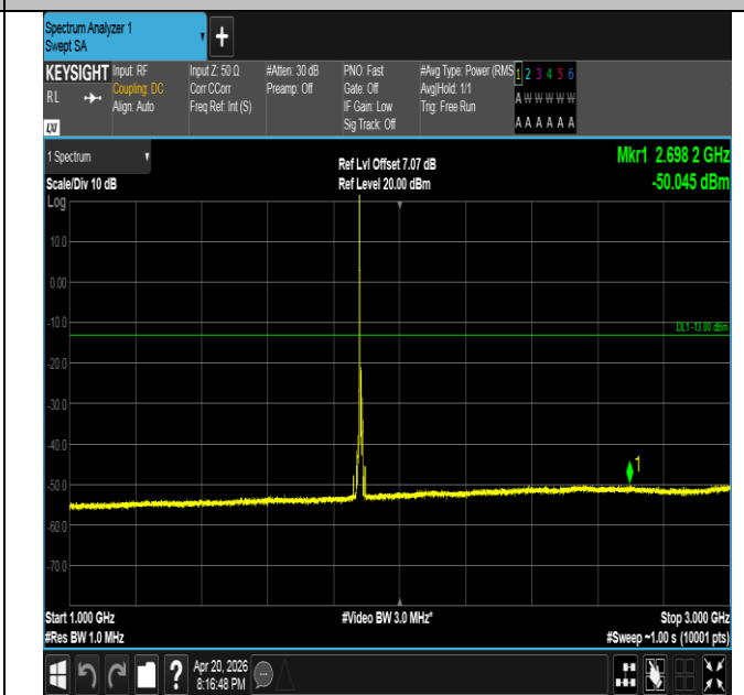
Band25-10MHz-QPSK-26365-1RB#0-1000~3000-PASS
