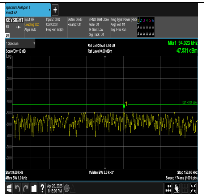
Band25-10MHz-QPSK-26365-1RB#49-0.009~0.15-PASS
