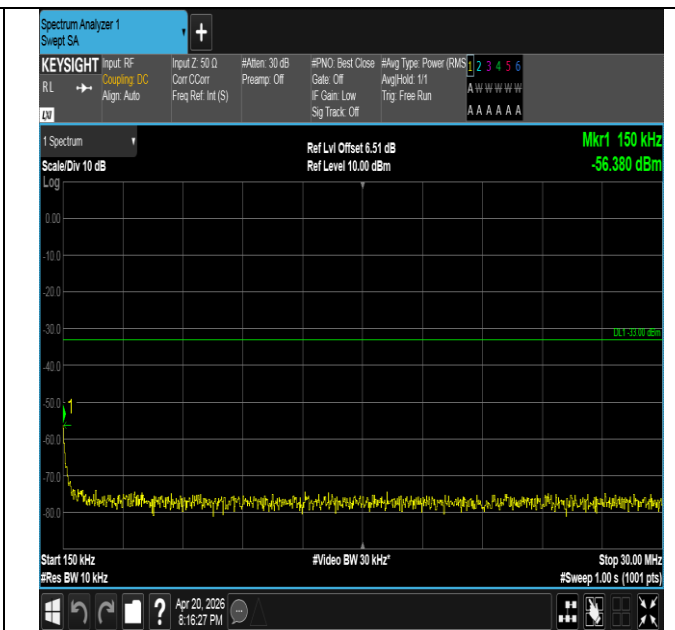
Band25-10MHz-QPSK-26365-1RB#0-0.15~30-PASS
