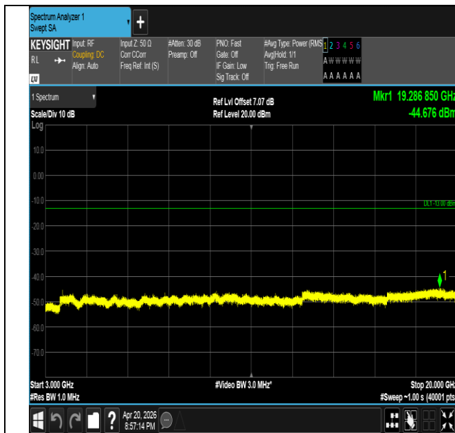
Band25-15MHz-QPSK-26115-1RB#0-3000~20000-PASS
