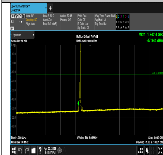
Band25-20MHz-QPSK-26140-1RB#99-1000~3000-PASS
