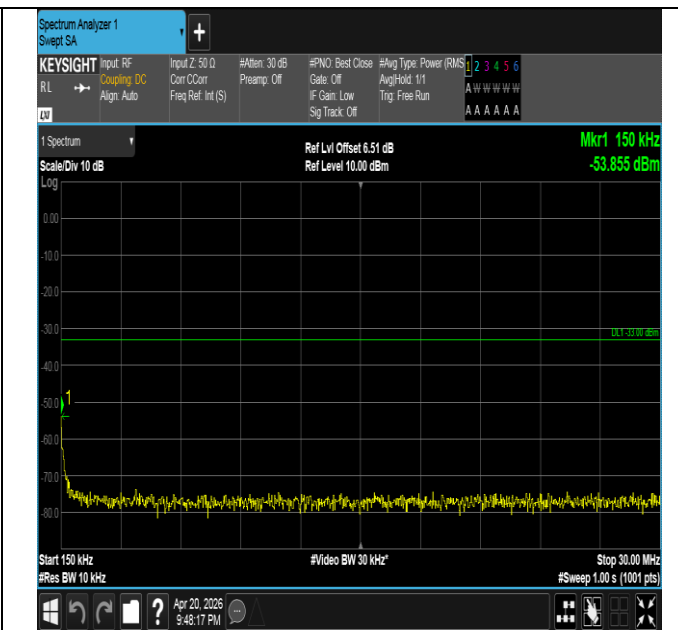
Band25-20MHz-QPSK-26365-1RB#0-0.15~30-PASS
