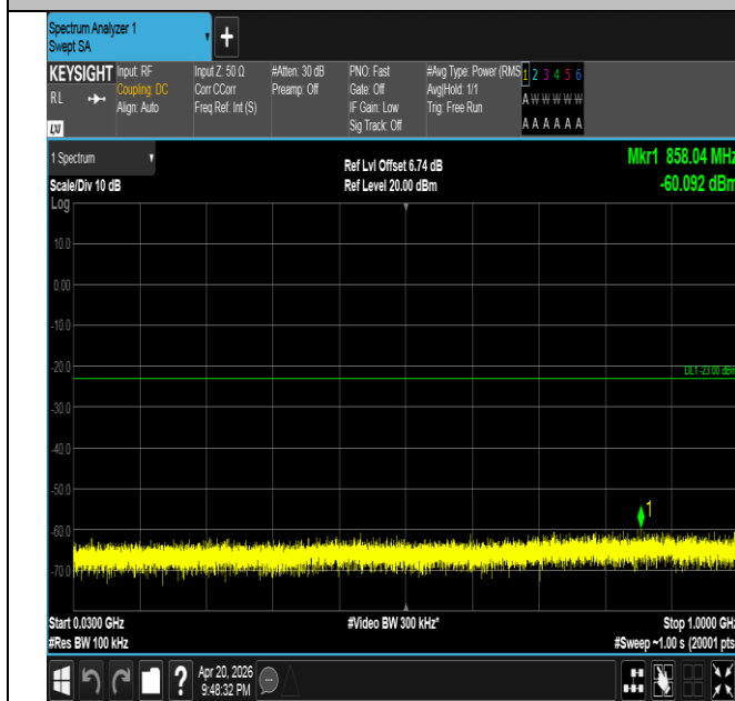
Band25-20MHz-QPSK-26365-1RB#0-30~1000-PASS
