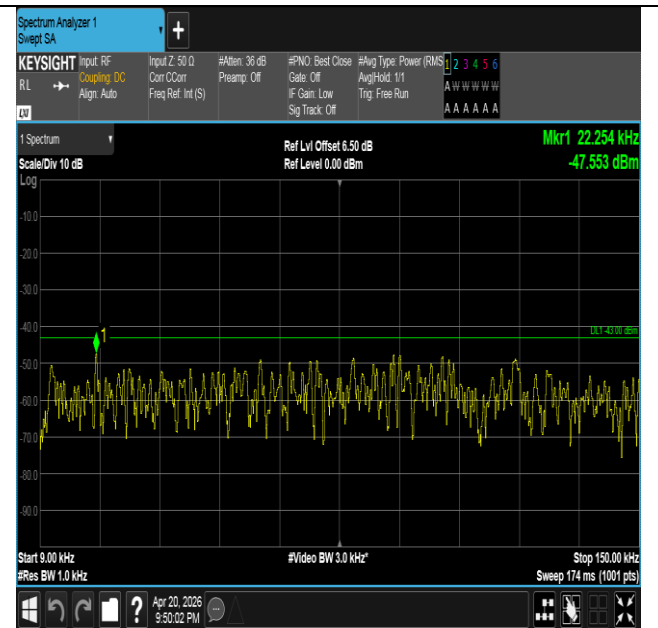
Band25-20MHz-QPSK-26365-1RB#99-0.009~0.15-PASS
