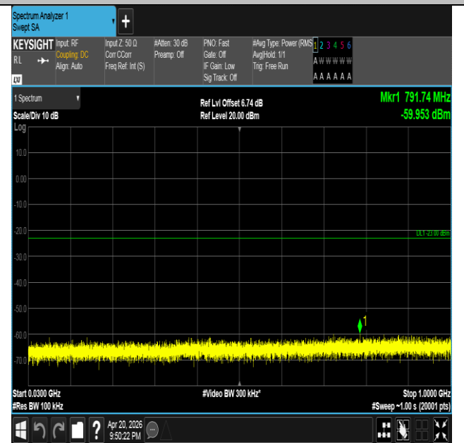
Band25-20MHz-QPSK-26365-1RB#99-30~1000-PASS
