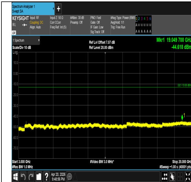
Band25-20MHz-QPSK-26365-1RB#0-3000~20000-PASS
