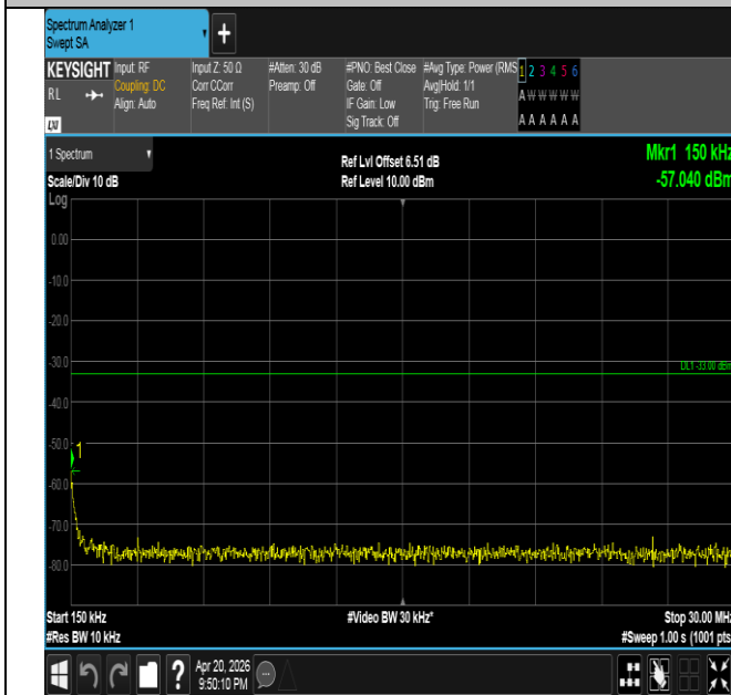
Band25-20MHz-QPSK-26365-1RB#99-0.15~30-PASS
