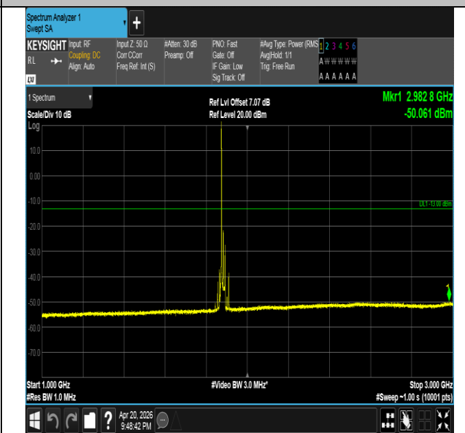
Band25-20MHz-QPSK-26365-1RB#0-1000~3000-PASS
