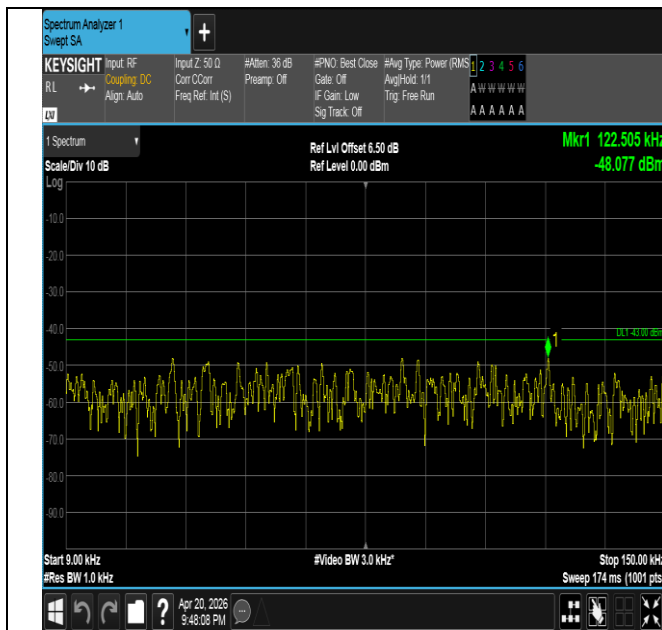
Band25-20MHz-QPSK-26365-1RB#0-0.009~0.15-PASS
