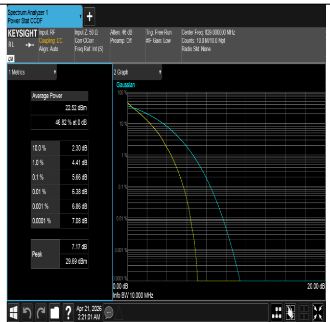
Band26(824-849)-10MHz-QPSK-26840-50RB#0-PASS
