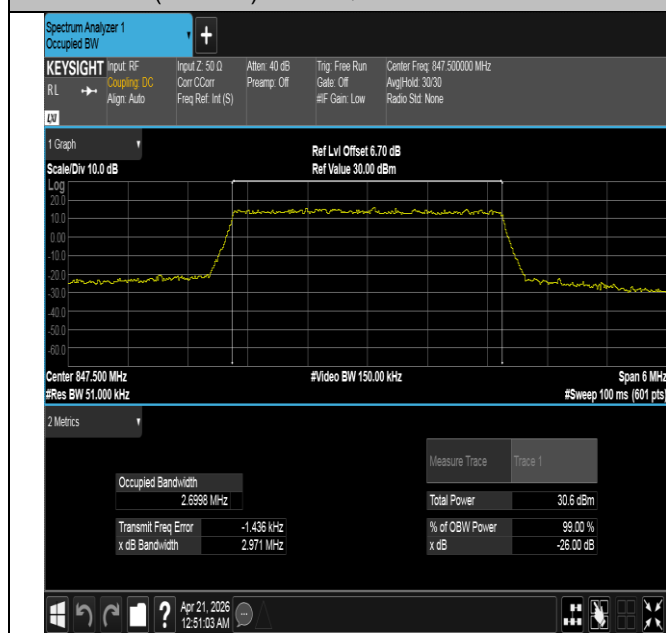
Band26(824-849)-3MHz-QPSK-27025-15RB#0-PASS
