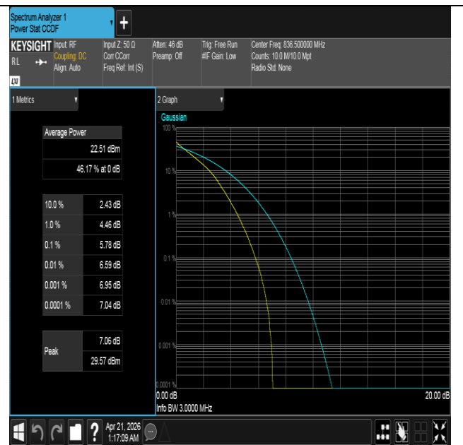
Band26(824-849)-3MHz-QPSK-26915-15RB#0-PASS
