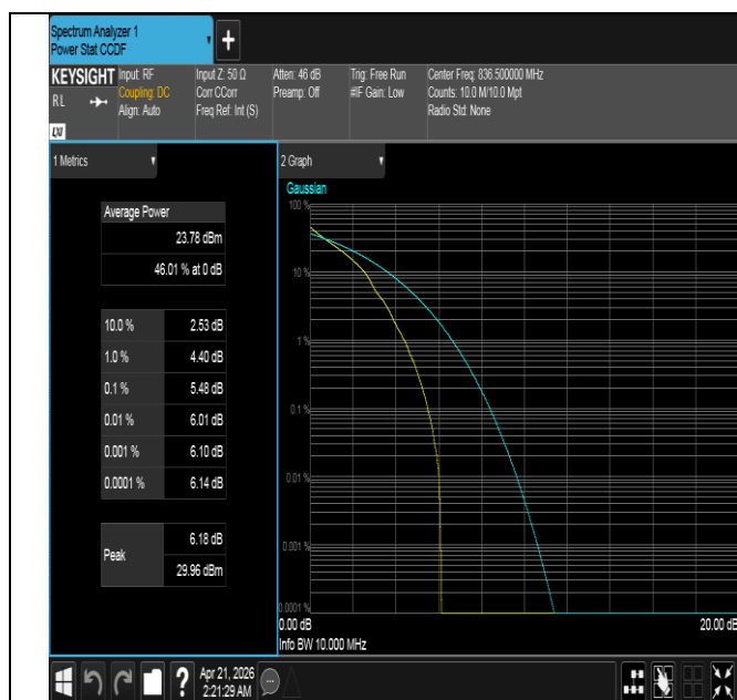
Band26(824-849)-10MHz-QPSK-26915-1RB#0-PASS
