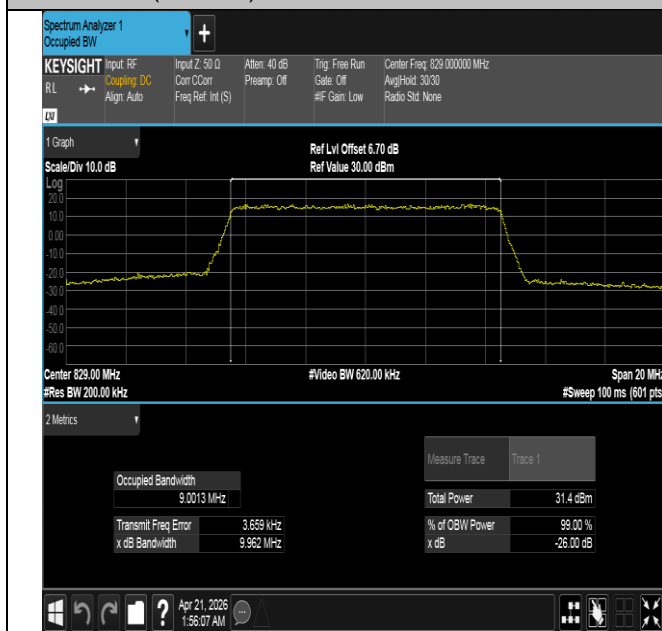
Band26(824-849)-10MHz-QPSK-26840-50RB#0-PASS
