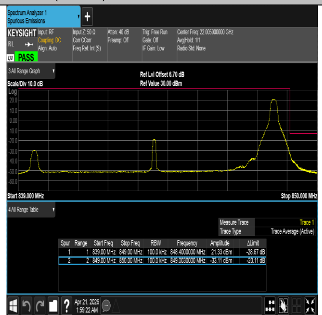
Band26(824-849)-10MHz-QPSK-26990-1RB#49-PASS
