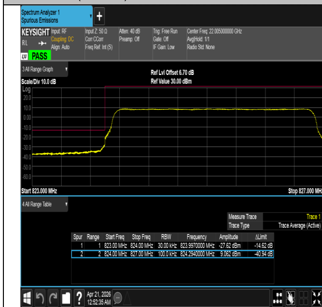
Band26(824-849)-3MHz-QPSK-26805-15RB#0-PASS
