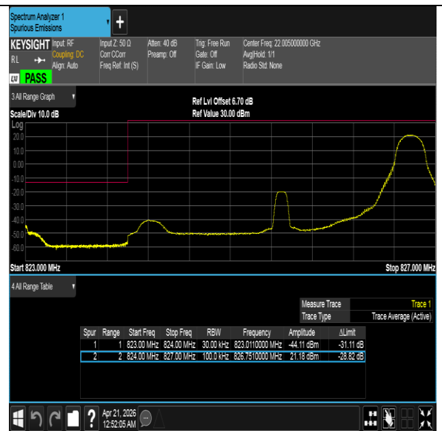
Band26(824-849)-3MHz-QPSK-26805-1RB#14-PASS
