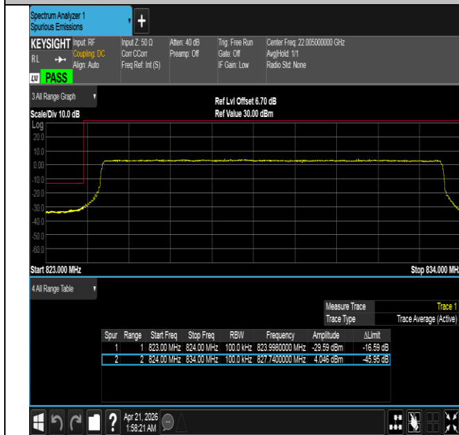
Band26(824-849)-10MHz-QPSK-26840-50RB#0-PASS
