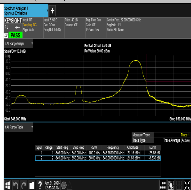
Band26(824-849)-3MHz-QPSK-27025-1RB#14-PASS
