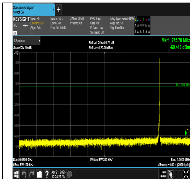
Band26(824-849)-1.4MHz-QPSK-26797-6RB#0-30~1000-PAS
