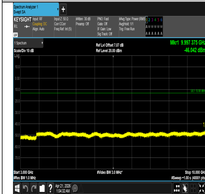
Band26(824-849)-3MHz-QPSK-26915-15RB#0-3000~10000-
