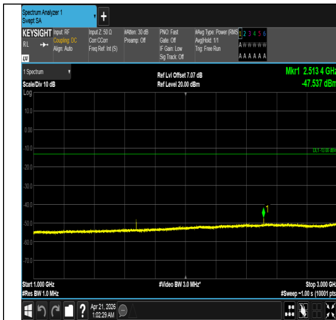
Band26(824-849)-3MHz-QPSK-26915-1RB#14-1000~3000-P
