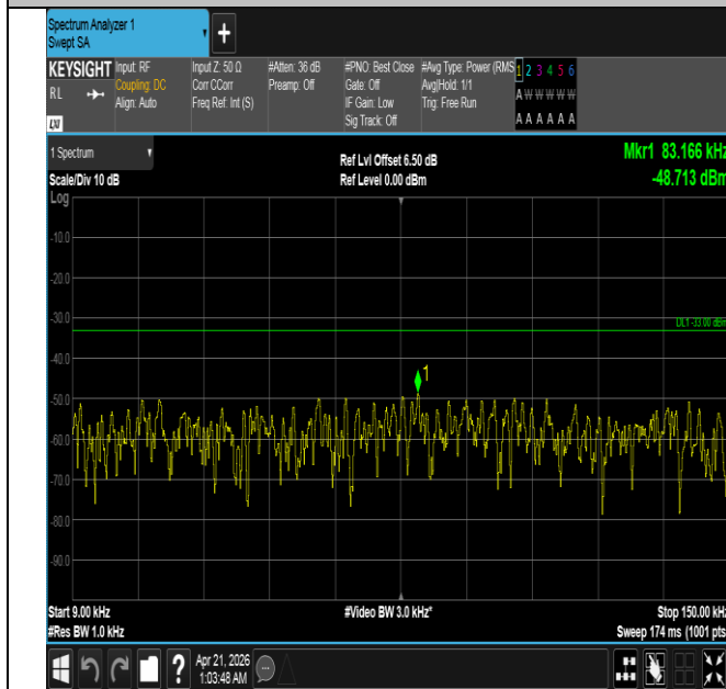
Band26(824-849)-3MHz-QPSK-26915-15RB#0-0.009~0.15-P
