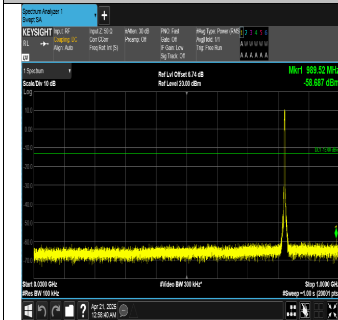
Band26(824-849)-3MHz-QPSK-26805-15RB#0-30~1000-PAS
