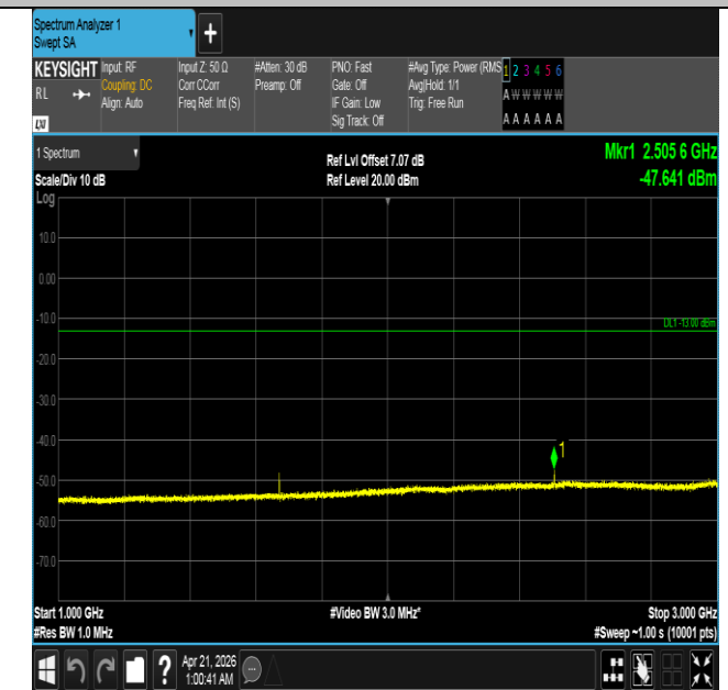
Band26(824-849)-3MHz-QPSK-26915-1RB#0-1000~3000-PA SS
