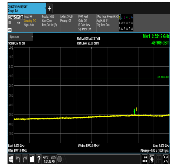
Band26(824-849)-3MHz-QPSK-26915-15RB#0-1000~3000-P
