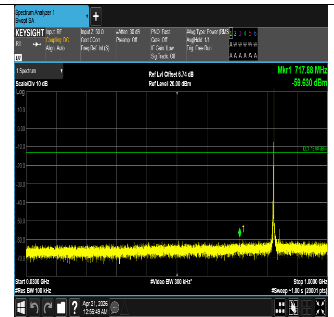
Band26(824-849)-3MHz-QPSK-26805-1RB#14-30~1000-PAS
