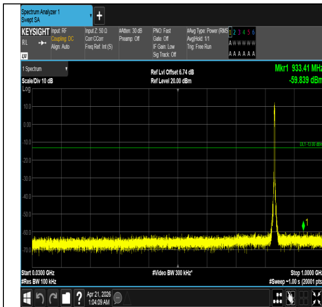
Band26(824-849)-3MHz-QPSK-26915-15RB#0-30~1000-PAS
