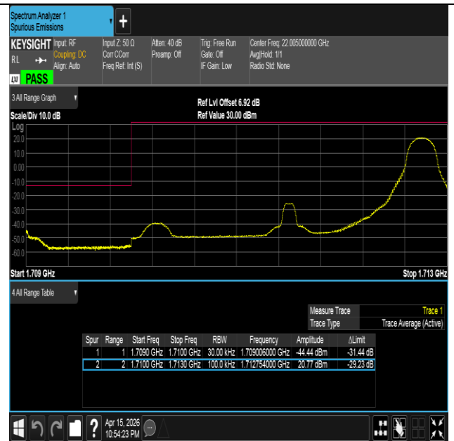
Band4-3MHz-QPSK-19965-1RB#14-PASS
