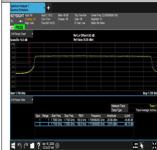
Band4-10MHz-QPSK-20000-50RB#0-PASS
