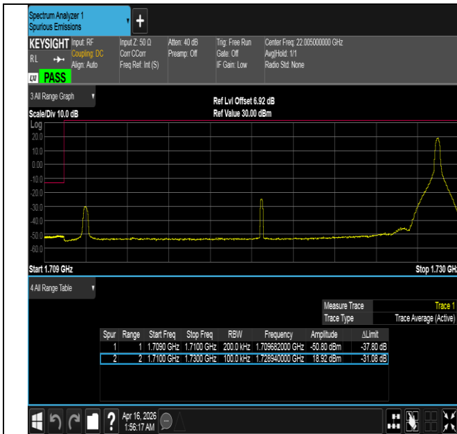
Band4-20MHz-16QAM-20050-1RB#99-PASS
