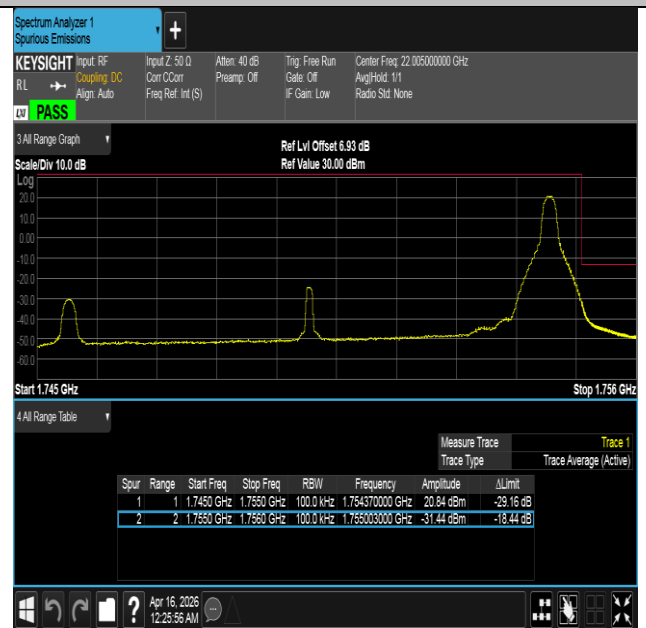
Band4-10MHz-QPSK-20350-1RB#49-PASS
