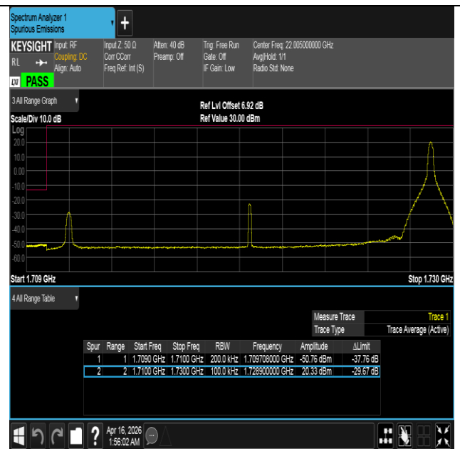
Band4-20MHz-QPSK-20050-1RB#99-PASS
