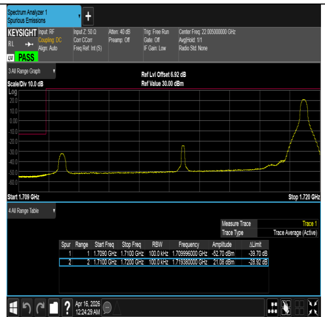
Band4-10MHz-QPSK-20000-1RB#49-PASS
