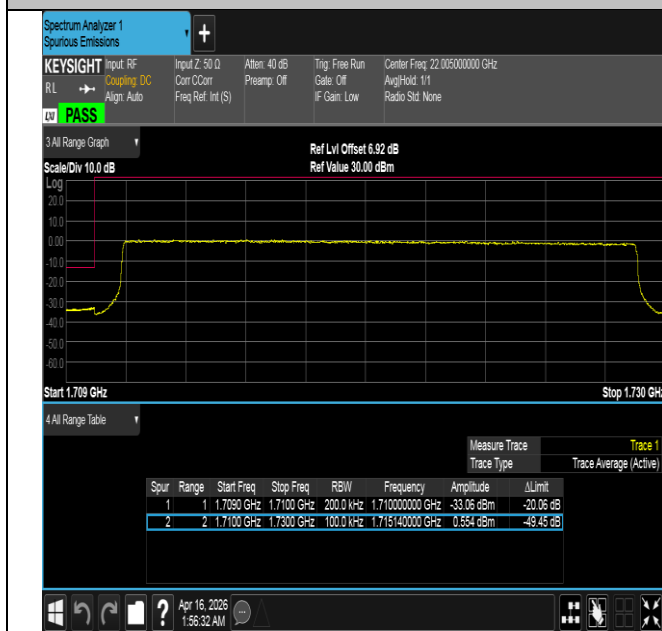
Band4-20MHz-QPSK-20050-100RB#0-PASS
