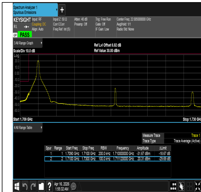
Band4-20MHz-QPSK-20050-1RB#0-PASS
