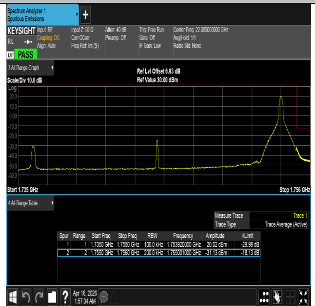
Band4-20MHz-QPSK-20300-1RB#99-PASS
