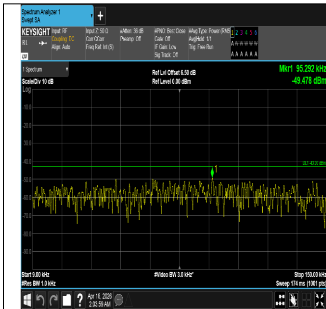
Band4-20MHz-QPSK-20175-1RB#0-0.009~0.15-PASS
