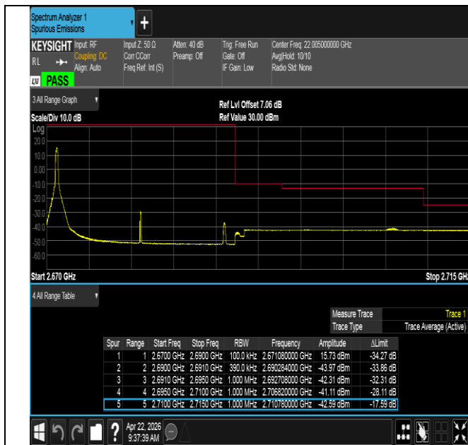
Band41-20MHz-QPSK-41490-1RB#0-PASS
