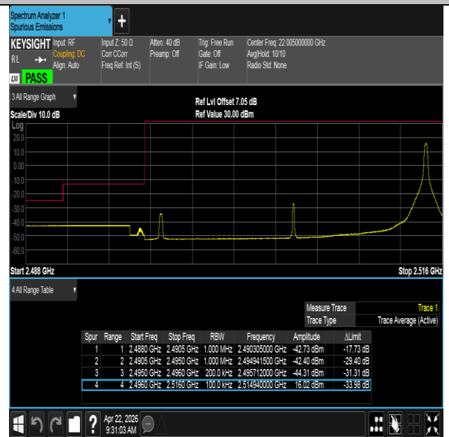
Band41-20MHz-QPSK-39750-1RB#99-PASS
