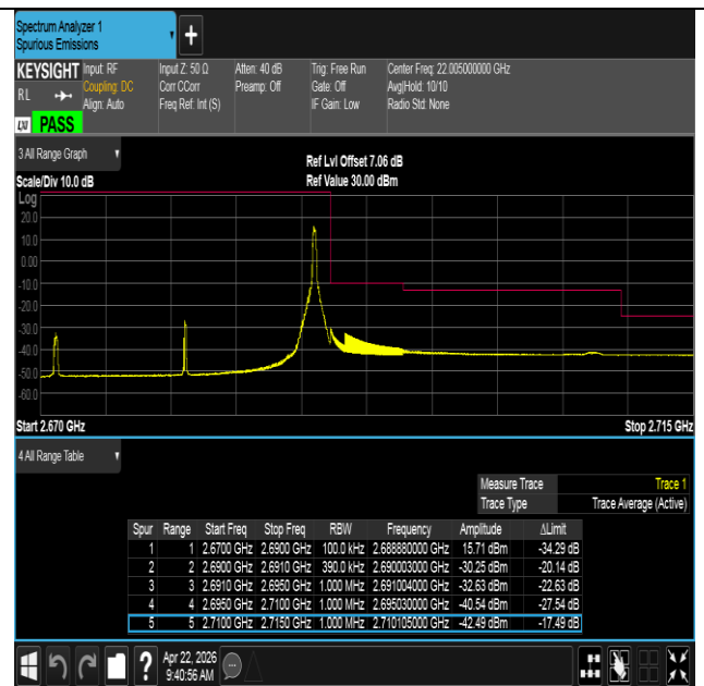
Band41-20MHz-QPSK-41490-1RB#99-PASS
