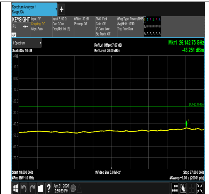
Band41-5MHz-16QAM-41565-1RB#0-18000~27000-PASS
