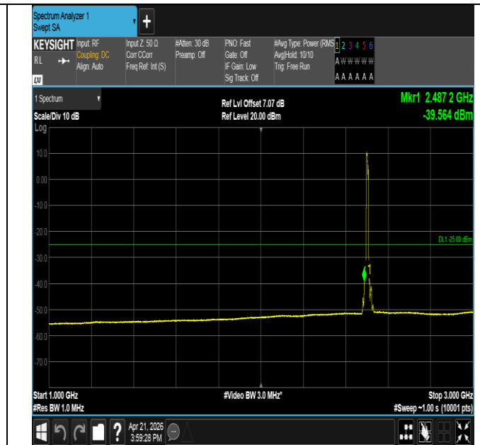
Band41-10MHz-QPSK-39700-50RB#0-1000~3000-PASS
