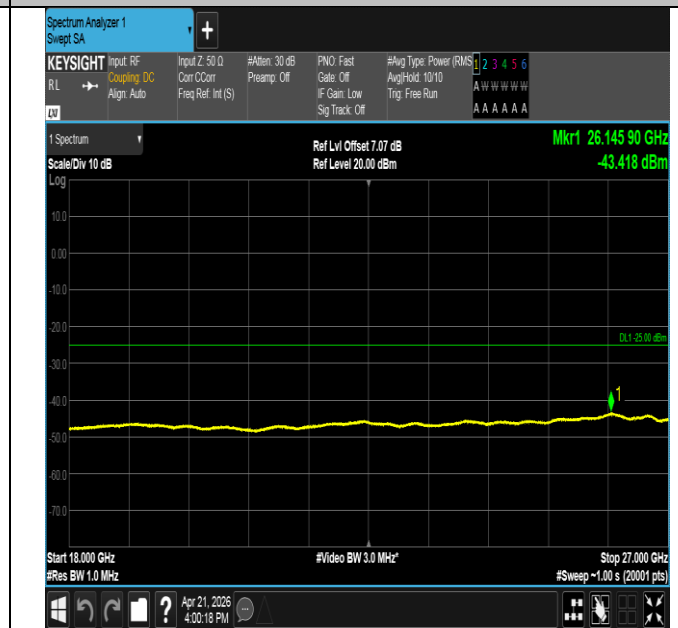
Band41-10MHz-QPSK-39700-50RB#0-18000~27000-PASS
