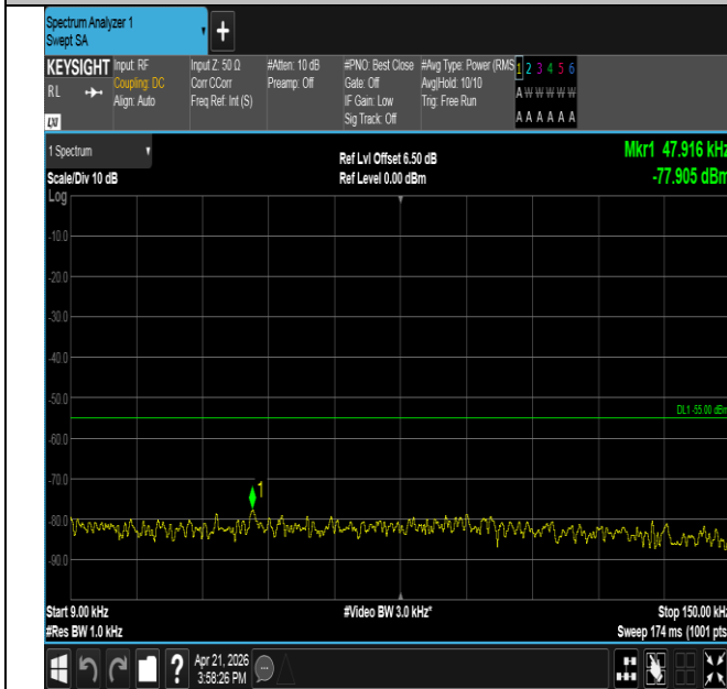
Band41-10MHz-QPSK-39700-50RB#0-0.009~0.15-PASS
