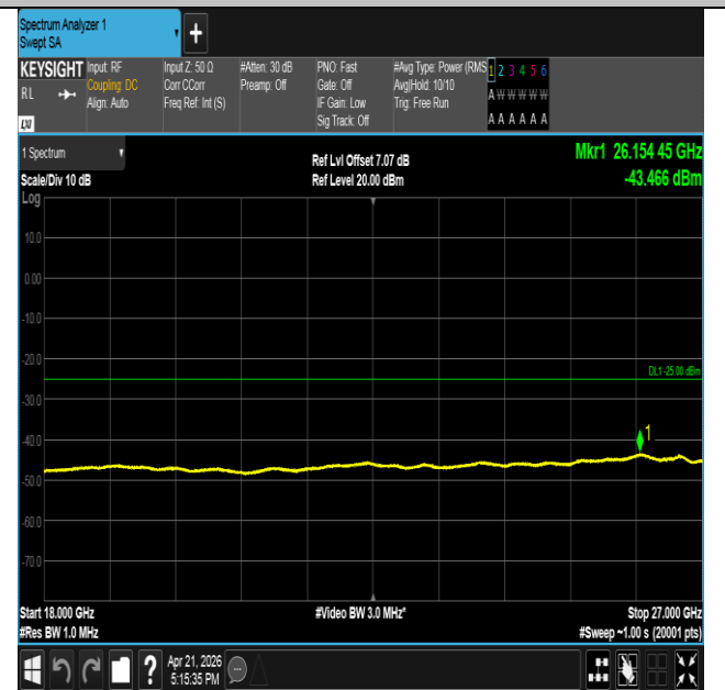
Band41-15MHz-QPSK-39725-1RB#0-18000~27000-PASS
