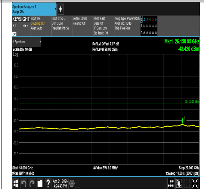
Band41-10MHz-QPSK-41540-50RB#0-18000~27000-PASS
