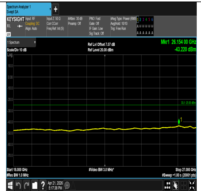
Band41-15MHz-16QAM-39725-1RB#0-18000~27000-PASS
