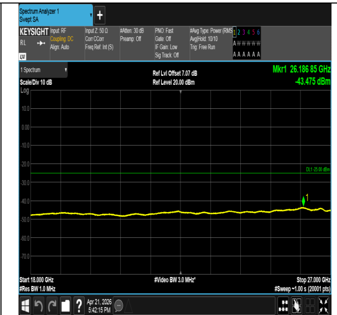
Band41-15MHz-16QAM-41515-1RB#0-18000~27000-PASS
