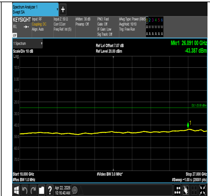
Band41-20MHz-QPSK-41490-1RB#99-18000~27000-PASS
