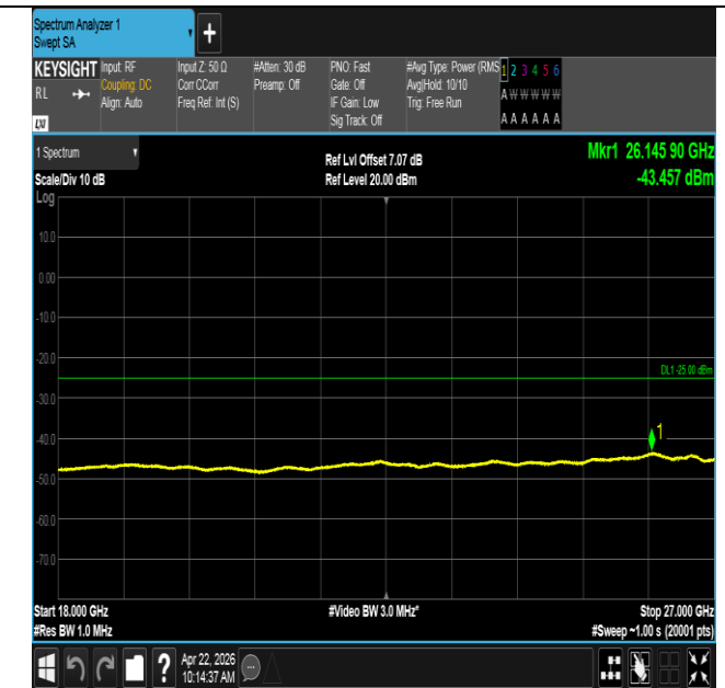
Band41-20MHz-16QAM-41490-1RB#0-18000~27000-PASS
