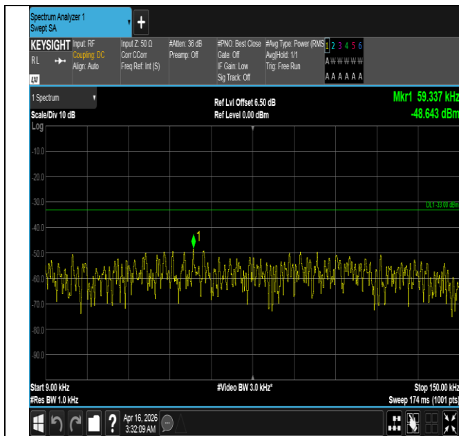
Band5-3MHz-QPSK-20635-1RB#0-0.009~0.15-PASS
