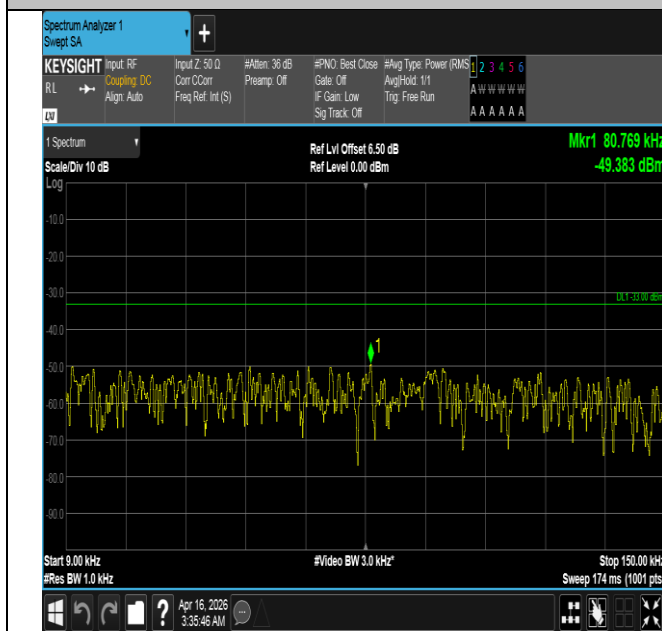
Band5-3MHz-QPSK-20635-15RB#0-0.009~0.15-PASS
