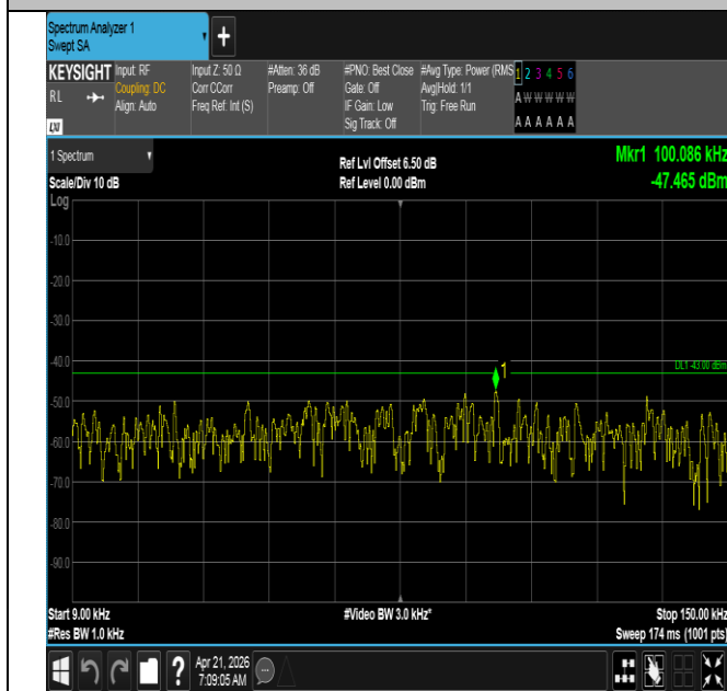
Band66-20MHz-QPSK-132572-1RB#0-0.009~0.15-PASS
