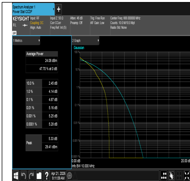
Band71-10MHz-QPSK-133172-1RB#0-PASS
