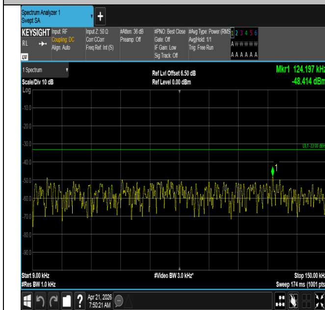
Band71-5MHz-QPSK-133147-25RB#0-0.009~0.15-PASS
