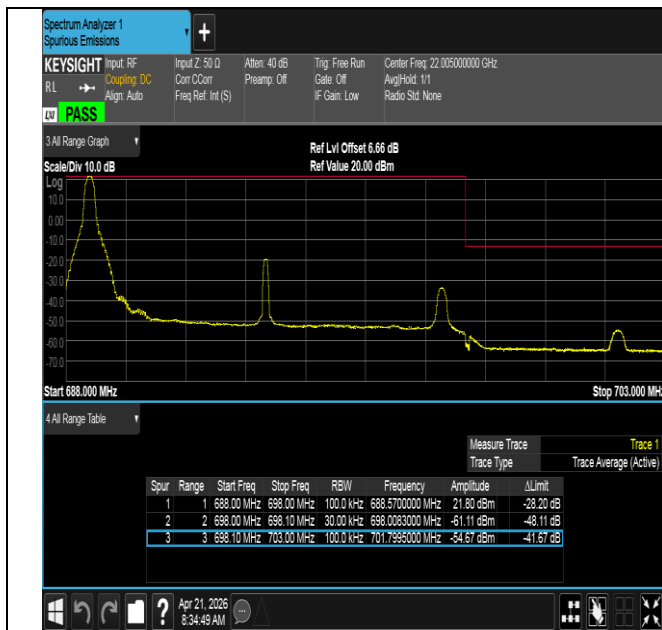
Band71-10MHz-QPSK-133422-1RB#0-PASS
