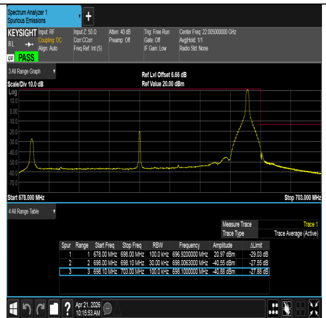
Band71-20MHz-QPSK-133372-1RB#99-PASS
