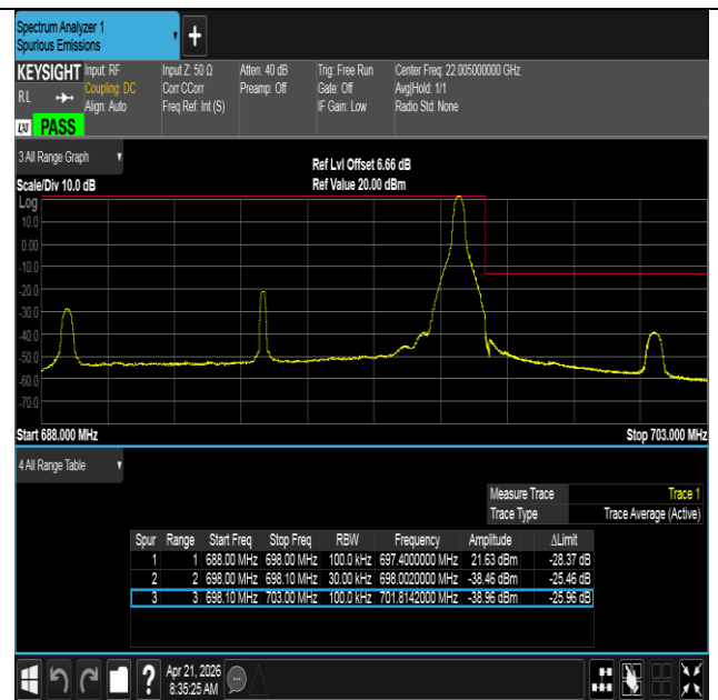
Band71-10MHz-QPSK-133422-1RB#49-PASS
