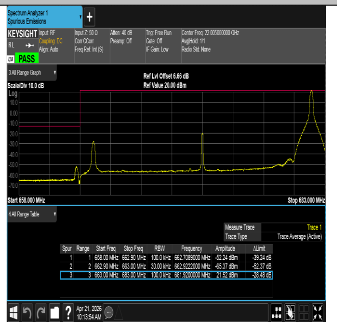
Band71-20MHz-QPSK-133222-1RB#99-PASS
