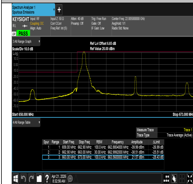
Band71-10MHz-QPSK-133172-1RB#0-PASS
