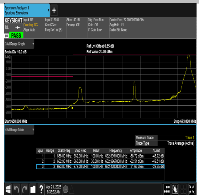
Band71-10MHz-QPSK-133172-1RB#49-PASS
