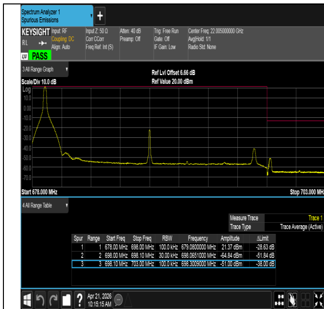
Band71-20MHz-QPSK-133372-1RB#0-PASS
