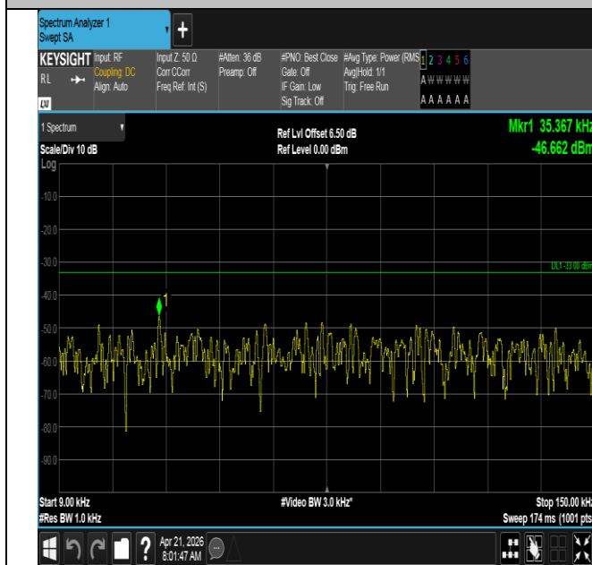
Band71-5MHz-QPSK-133447-25RB#0-0.009~0.15-PASS
