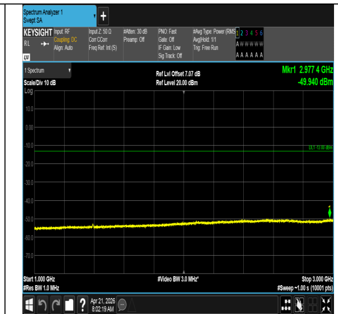
Band71-5MHz-QPSK-133447-25RB#0-1000~3000-PASS
