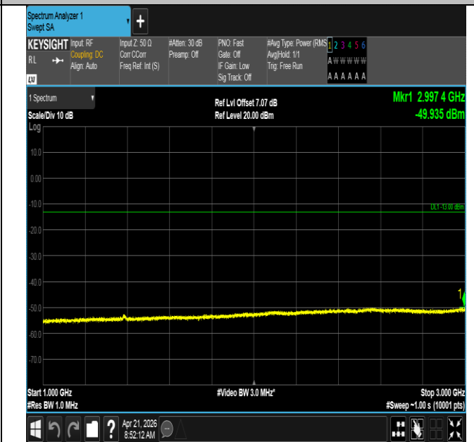
Band71-10MHz-QPSK-133422-50RB#0-1000~3000-PASS
