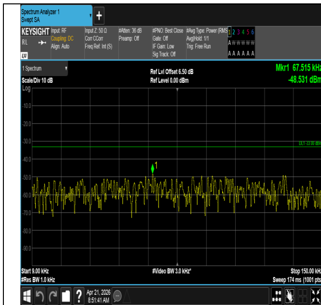
Band71-10MHz-QPSK-133422-50RB#0-0.009~0.15-PASS
