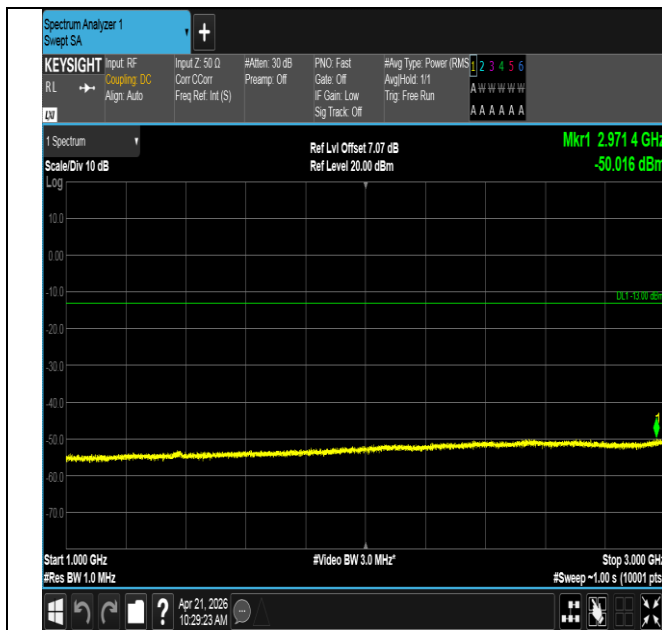
Band71-20MHz-QPSK-133372-100RB#0-1000~3000-PASS
