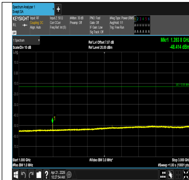
Band71-20MHz-QPSK-133372-1RB#99-1000~3000-PASS
