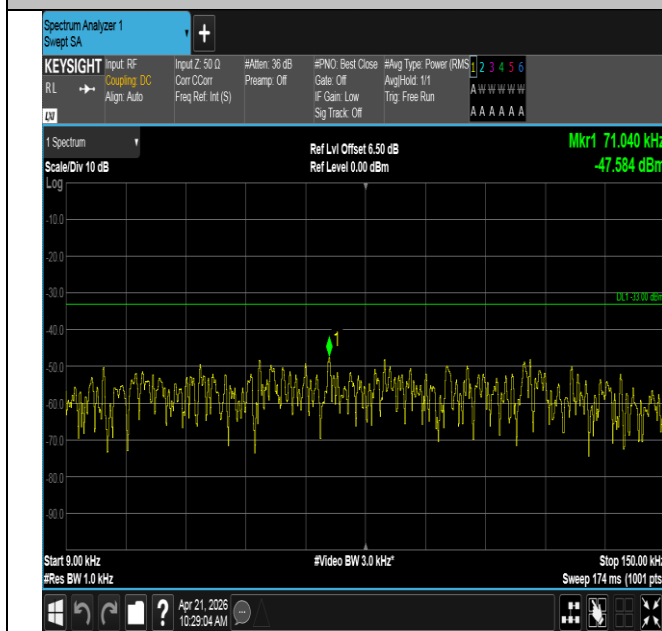
Band71-20MHz-QPSK-133372-100RB#0-0.009~0.15-PASS
