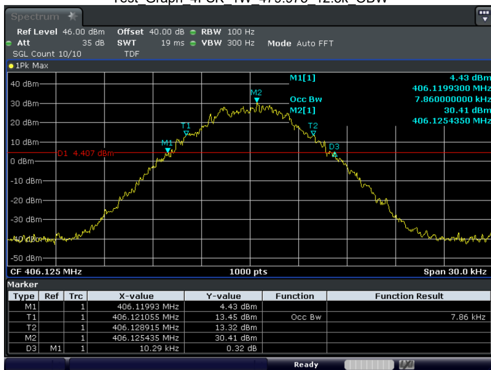
Test_Graph_4FSK_4W_406.125_12.5k_OBW
