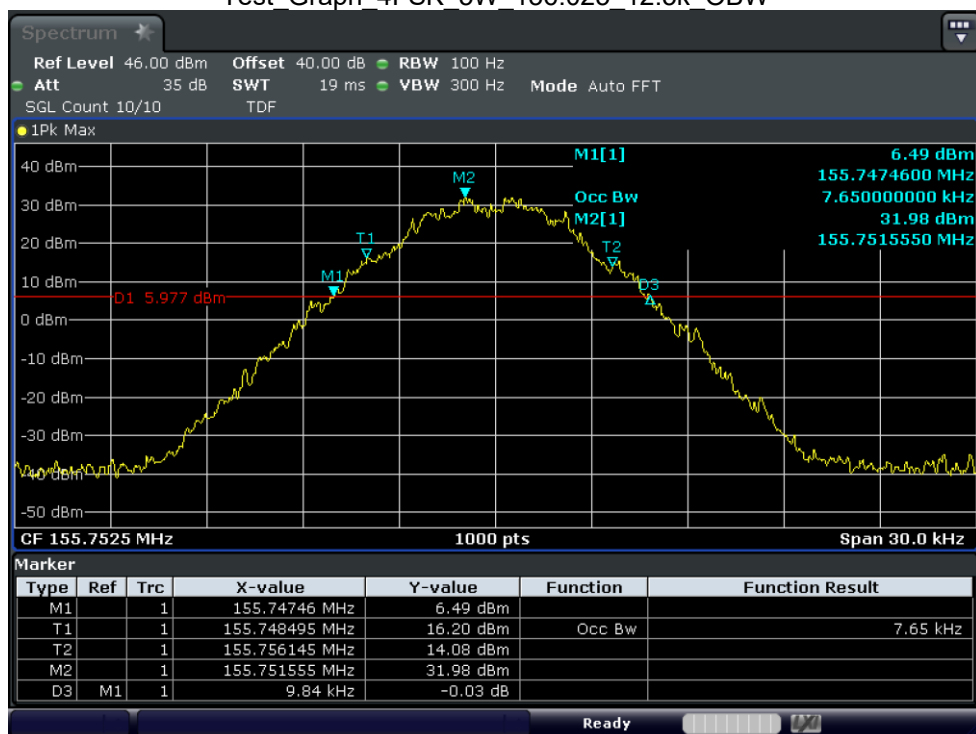
Test_Graph_4FSK_5W_155.7525_12.5k_OBW
