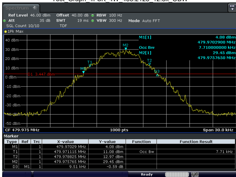
Test_Graph_4FSK_4W_479.975_12.5k_OBW
