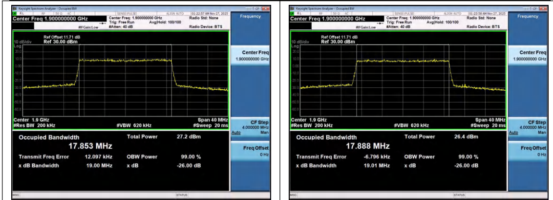
Band2-20MHz-QPSK-19100-100RB#0-PASS
