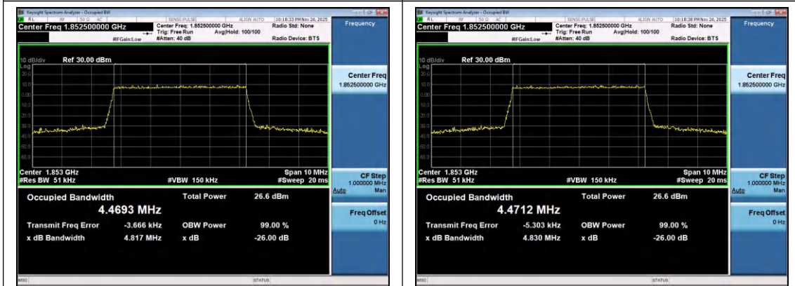
Band2-5MHz-QPSK-18625-25RB#0-PASS
