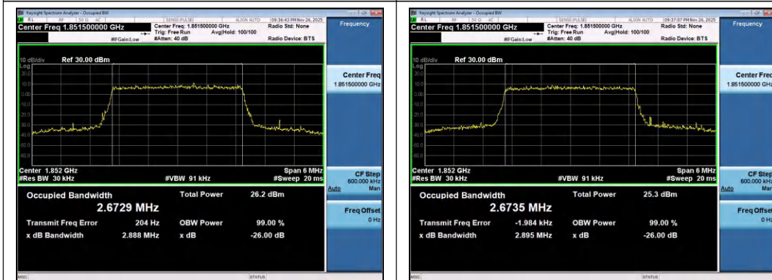
Band2-3MHz-QPSK-18615-15RB#0-PASS
