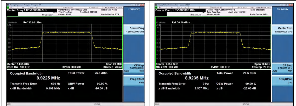
Band2-10MHz-QPSK-18650-50RB#0-PASS
