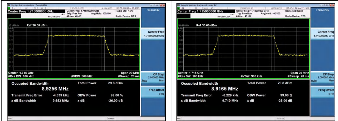
Band4-10MHz-QPSK-20000-50RB#0-PASS
