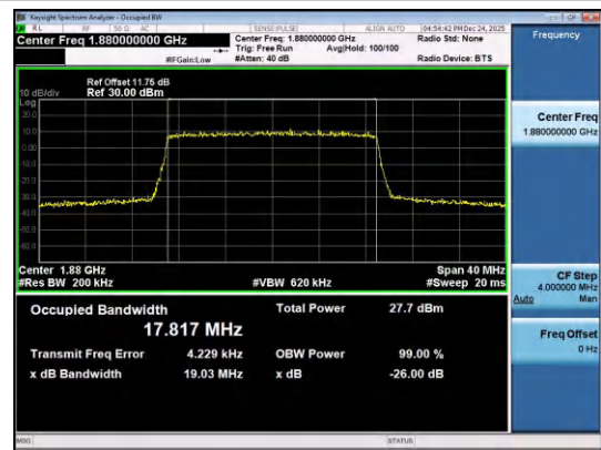
Band2-20MHz-QPSK-18900-100RB#0-PASS
