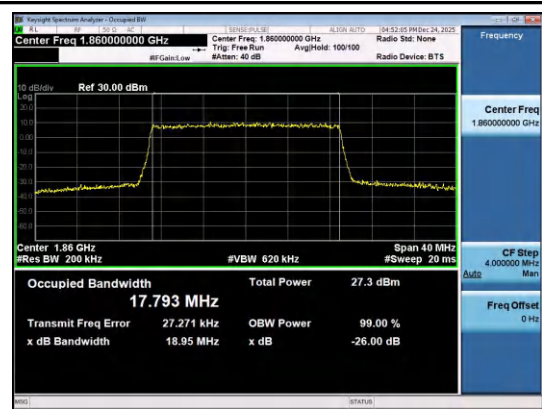
Band2-20MHz-QPSK-18700-100RB#0-PASS
