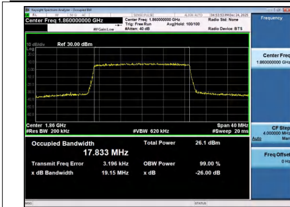
Band2-20MHz-16QAM-18700-100RB#0-PASS
