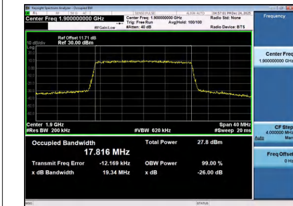
Band2-20MHz-QPSK-19100-100RB#0-PASS
