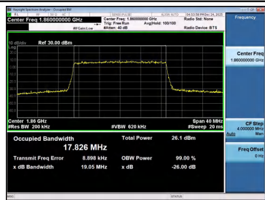
Band2-20MHz-16QAM-18700-100RB#0-PASS
