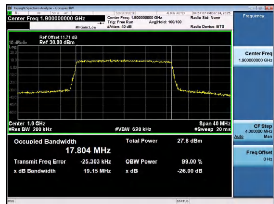
Band2-20MHz-QPSK-19100-100RB#0-PASS
