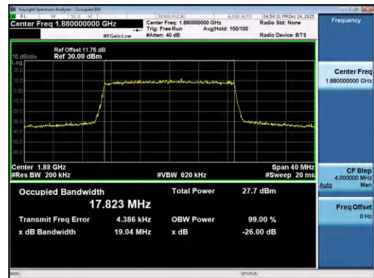
Band2-20MHz-QPSK-18900-100RB#0-PASS
