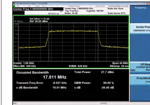
Band2-20MHz-QPSK-18900-100RB#0-PASS
