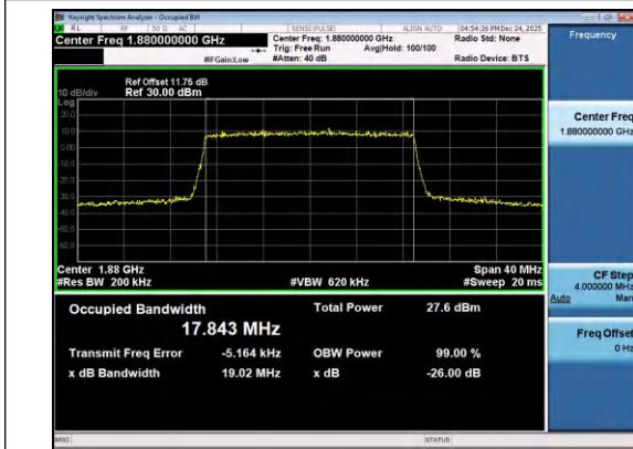
Band2-20MHz-QPSK-18900-100RB#0-PASS
