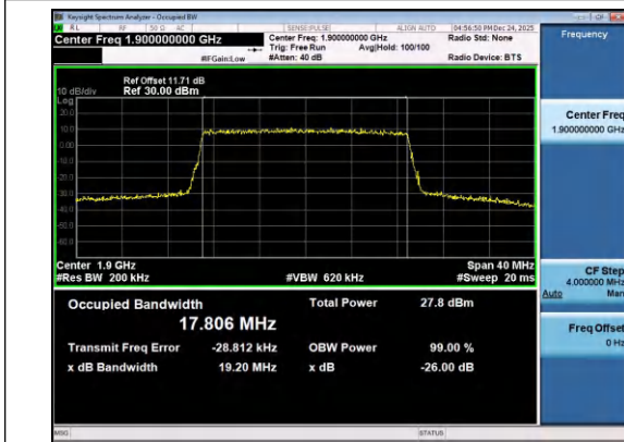
Band2-20MHz-QPSK-19100-100RB#0-PASS
