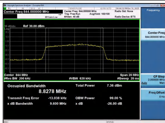
Band26(824-849)-10MHz-QPSK-26990-50RB#0-PAS
