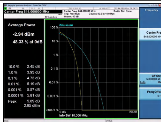
Band26(824-849)-10MHz-QPSK-26990-50RB#0-PASS
