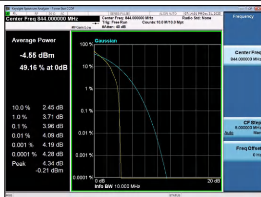
Band26(824-849)-10MHz-QPSK-26990-1RB#0-PASS
