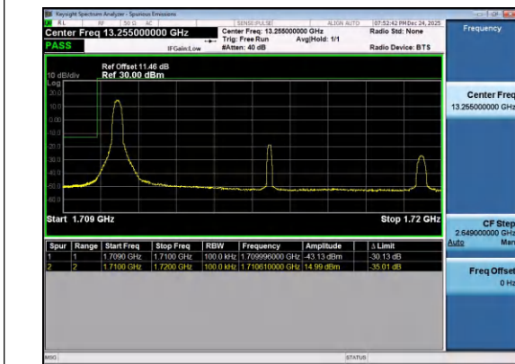
Band4-10MHz-QPSK-20000-1RB#0-PASS
