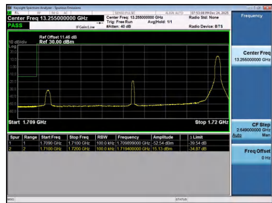
Band4-10MHz-QPSK-20000-1RB#49-PASS
