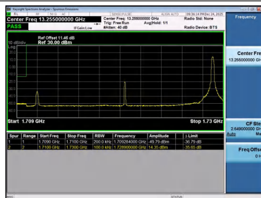
Band4-20MHz-QPSK-20050-1RB#99-PASS
