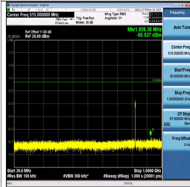
Band26(824-849)-3MHz-QPSK-26805-15RB#0-30~1000-P ASS
