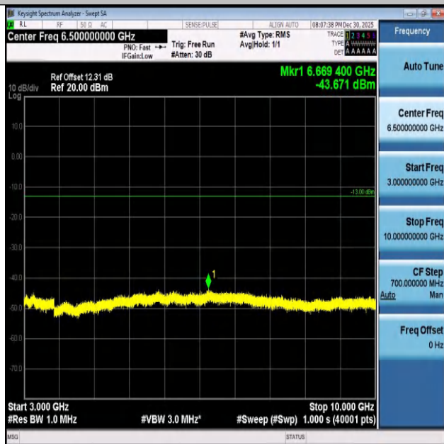
Band26(824-849)-3MHz-QPSK-26915-15RB#0-3000~100 00-PASS
