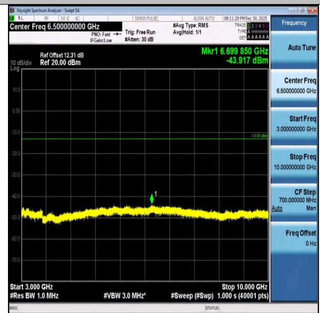
Band26(824-849)-3MHz-QPSK-27025-1RB#14-3000~100
