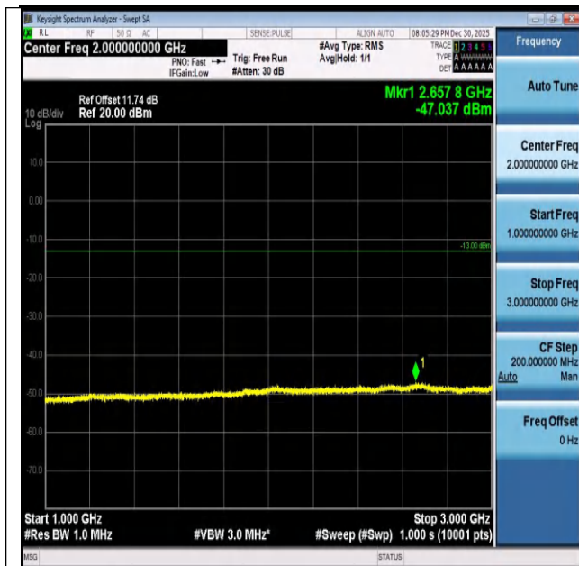
Band26(824-849)-3MHz-QPSK-26915-1RB#14-1000~300 0-PASS
