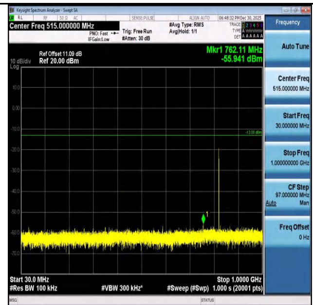
Band26(824-849)-1.4MHz-16QAM-26797-1RB#0-30~1000 -PASS
