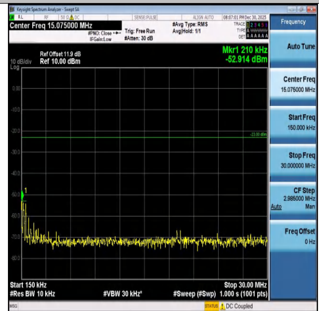
Band26(824-849)-3MHz-QPSK-26915-15RB#0-0.15~30-P ASS
