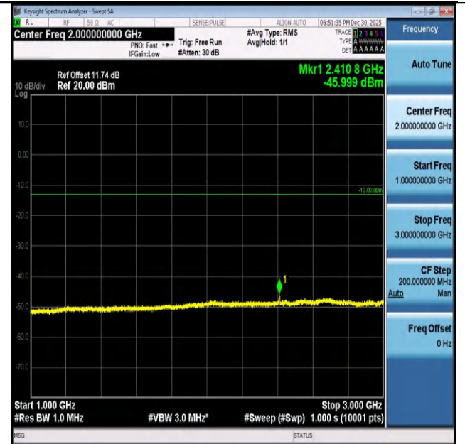
Band26(824-849)-1.4MHz-QPSK-26797-6RB#0-1000~300- 0-PASS
