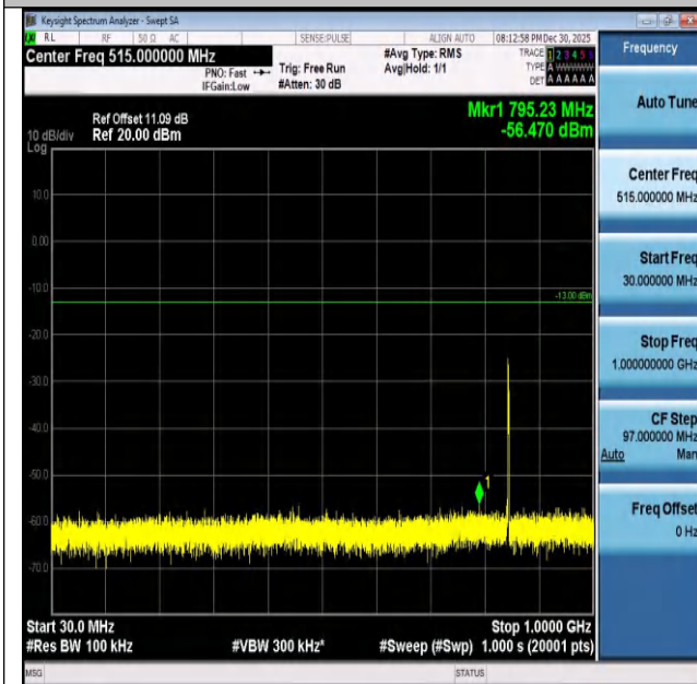
Band26(824-849)-3MHz-QPSK-27025-15RB#0-30~1000-P ASS
