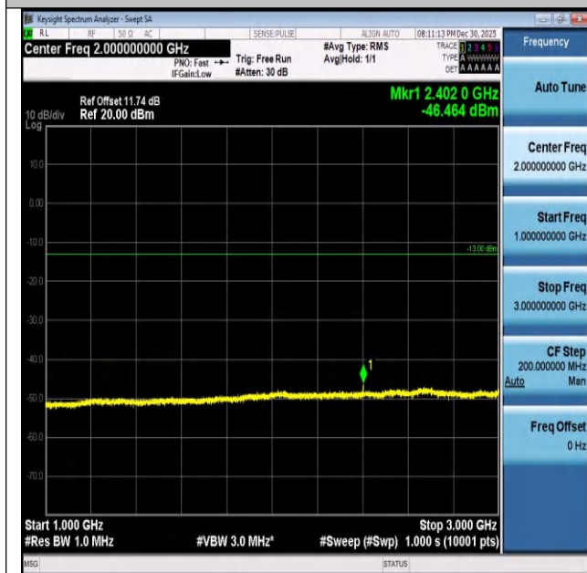
Band26(824-849)-3MHz-QPSK-27025-1RB#14-1000~300
