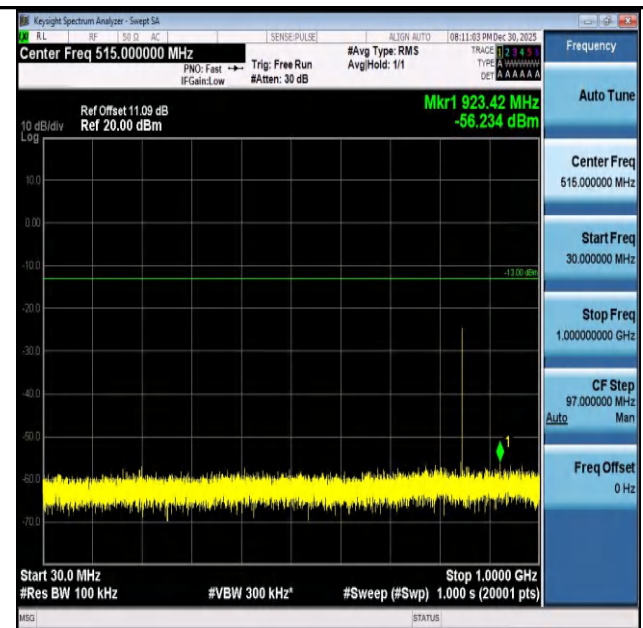
Band26(824-849)-3MHz-QPSK-27025-1RB#14-30~1000-P
