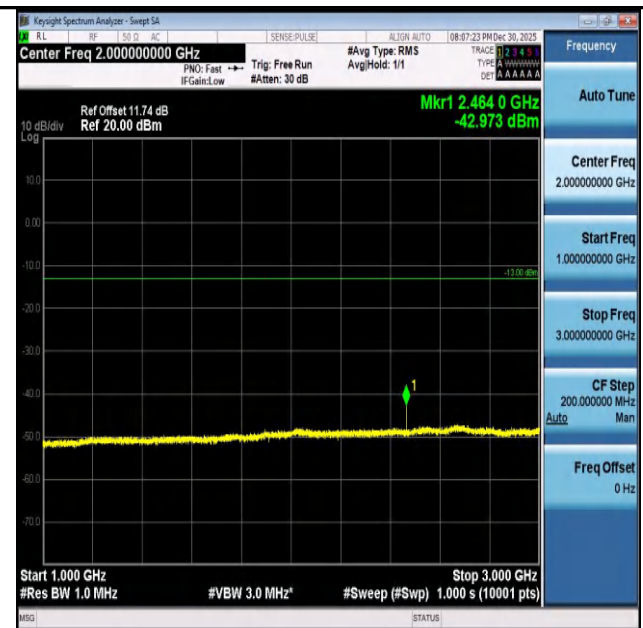
Band26(824-849)-3MHz-QPSK-26915-15RB#0-1000~300 0-PASS
