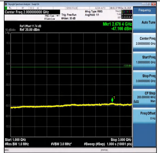
Band26(824-849)-3MHz-QPSK-26805-15RB#0-1000~300 0-PASS
