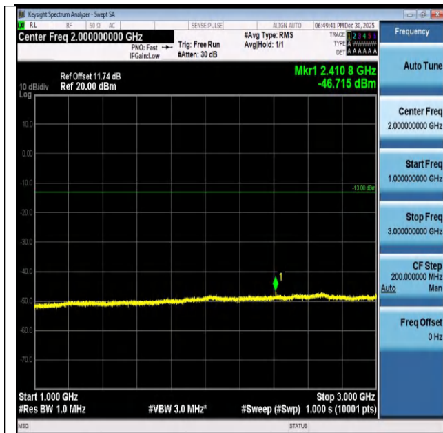
Band26(824-849)-1.4MHz-QPSK-26797-1RB#5-1000~300 0-PASS
