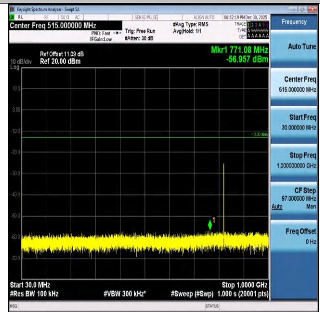
Band26(824-849)-1.4MHz-16QAM-26797-6RB#0-30~1000 -PASS
