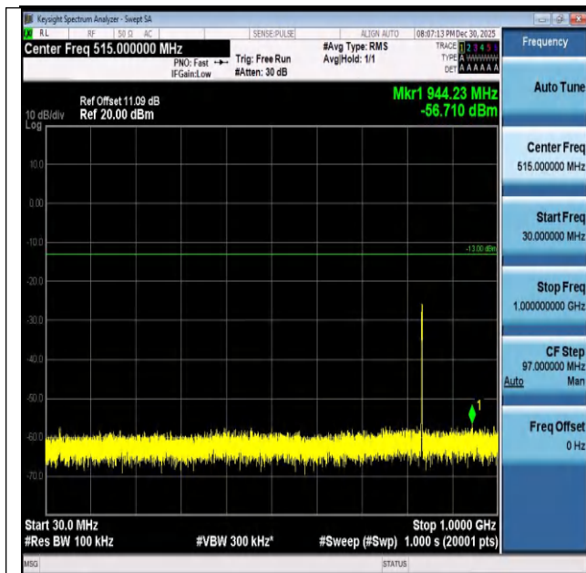
Band26(824-849)-3MHz-QPSK-26915-15RB#0-30~1000-P ASS
