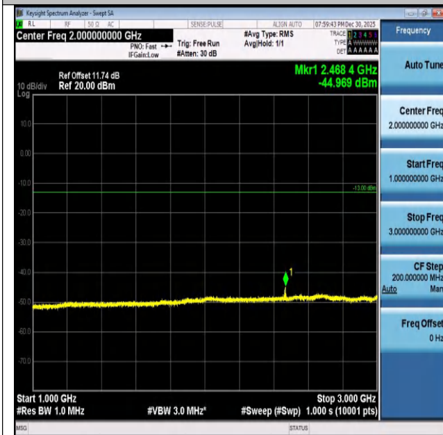
Band26(824-849)-3MHz-QPSK-26805-1RB#14-1000~300
