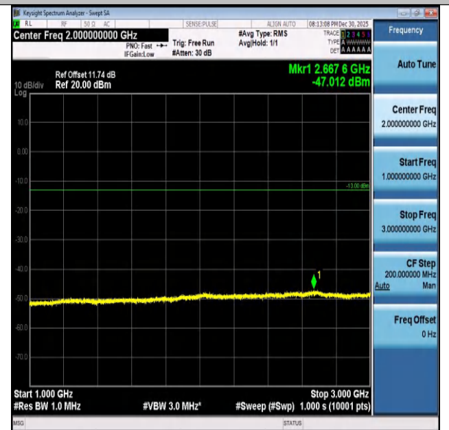
Band26(824-849)-3MHz-QPSK-27025-15RB#0-1000~300 0-PASS
