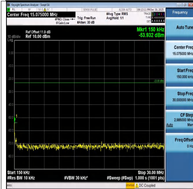
Band26(824-849)-10MHz-16QAM-26840-50RB#0-0.15~30 -PASS
