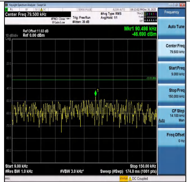
Band26(824-849)-10MHz-16QAM-26840-50RB#0-0.009~0 .15-PASS
