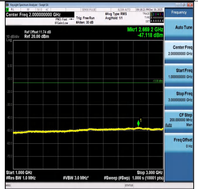
Band26(824-849)-10MHz-QPSK-26915-50RB#0-1000~3000-PASS
