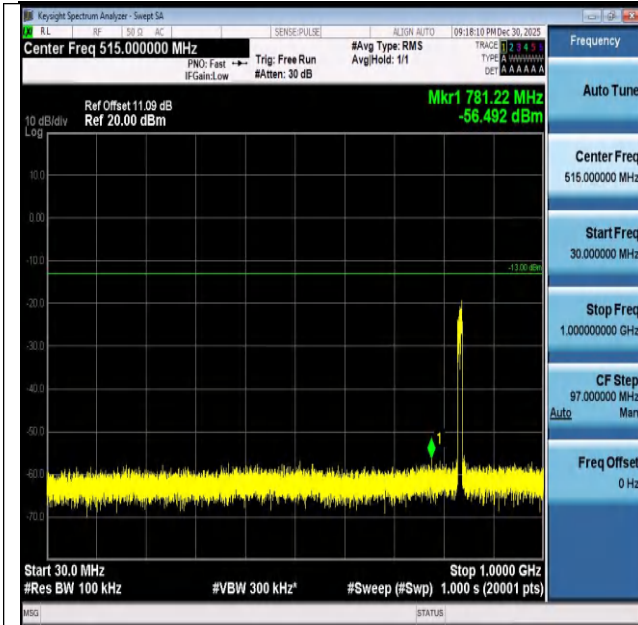
Band26(824-849)-10MHz-QPSK-26915-50RB#0-30~1000-PASS
