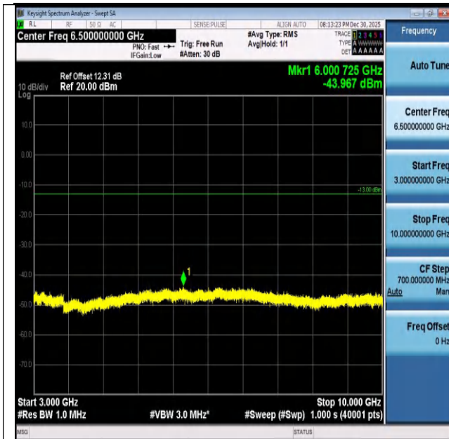
Band26(824-849)-3MHz-QPSK-27025-15RB#0-3000~100 00-PASS
