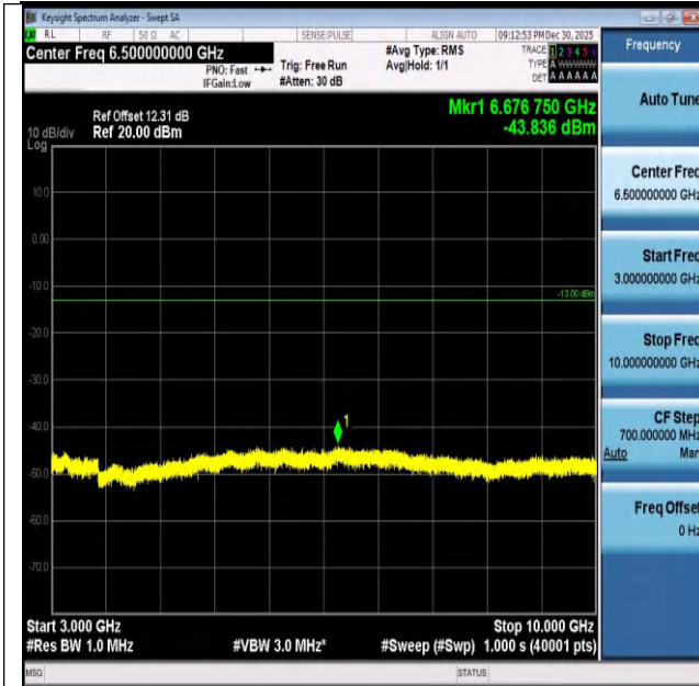
Band26(824-849)-10MHz-QPSK-26840-50RB#0-3000~10000-PASS
