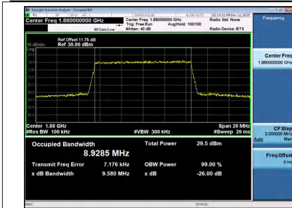
Band2-10MHz-QPSK-18900-50RB#0-PASS
