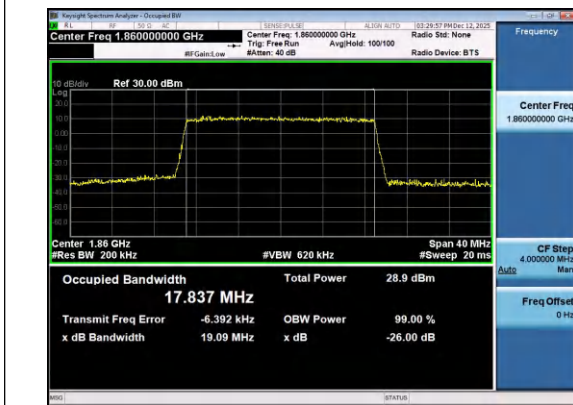
Band2-20MHz-16QAM-18700-100RB#0-PASS
