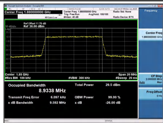
Band2-10MHz-QPSK-18900-50RB#0-PASS
