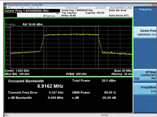
Band2-10MHz-QPSK-18650-50RB#0-PASS
