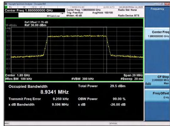
Band2-10MHz-QPSK-18900-50RB#0-PASS
