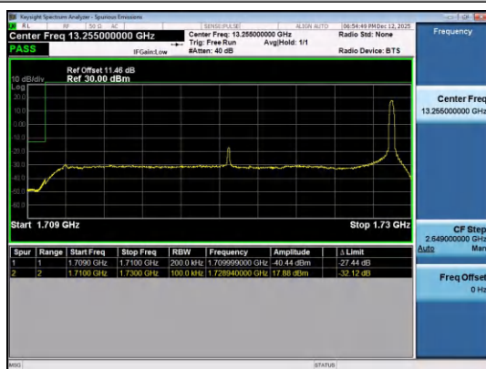
Band4-20MHz-16QAM-20050-1RB#99-PASS
