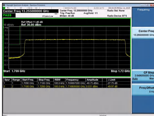
Band4-10MHz-QPSK-20000-50RB#0-PASS
