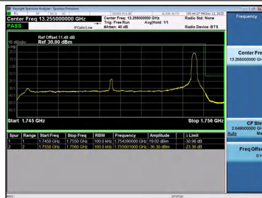
Band4-10MHz-QPSK-20350-1RB#49-PASS
