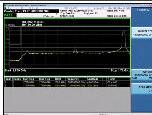
Band4-10MHz-QPSK-20000-1RB#49-PASS
