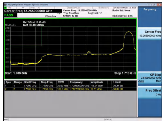
Band4-3MHz-QPSK-19965-1RB#14-PASS
