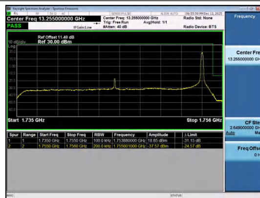
Band4-20MHz-QPSK-20300-1RB#99-PASS
