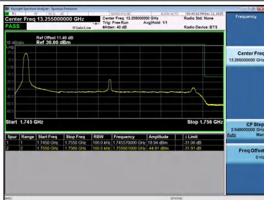
Band4-10MHz-QPSK-20350-1RB#0-PASS
