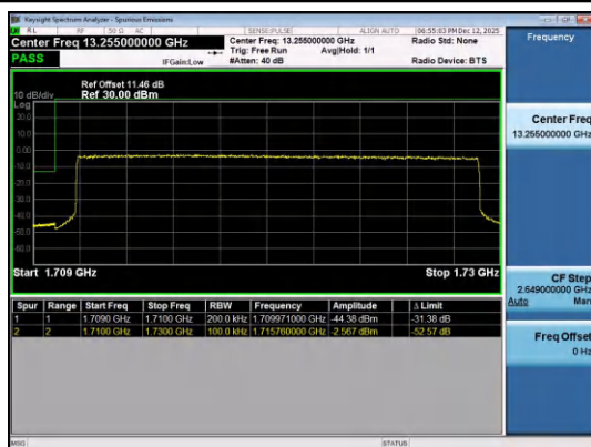
Band4-20MHz-QPSK-20050-100RB#0-PASS
