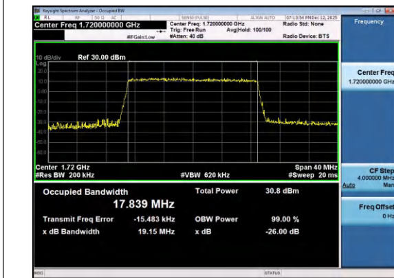
Band4-20MHz-QPSK-20050-100RB#0-PASS
