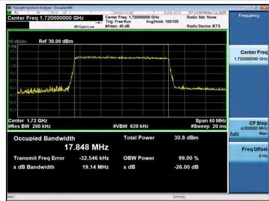
Band4-20MHz-QPSK-20050-100RB#0-PASS
