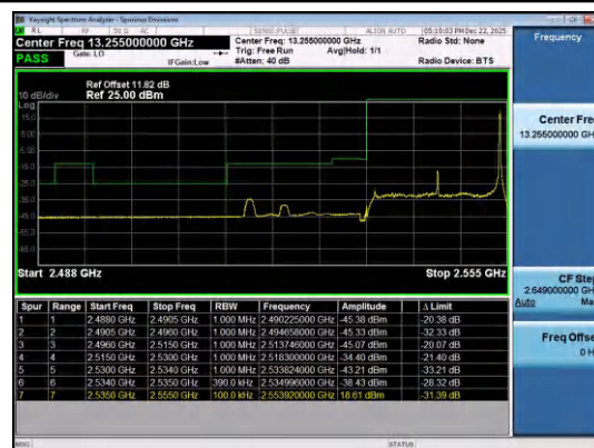
Band41(2535-2655)-20MHz-QPSK-40140-1RB#99-PA
