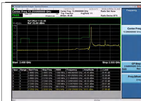
Band41(2535-2655)-20MHz-QPSK-40140-1RB#0-PA
