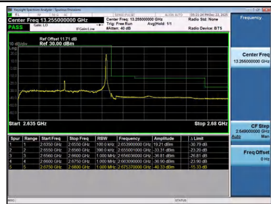
Band41(2535-2655)-20MHz-QPSK-41140-1RB#99-PAS
