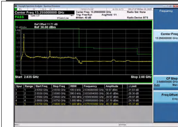
Band41(2535-2655)-20MHz-QPSK-41140-1RB#0-PAS
