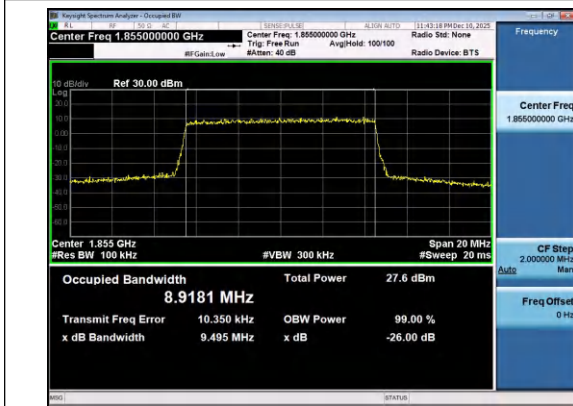
Band2-10MHz-QPSK-18650-50RB#0-PASS
