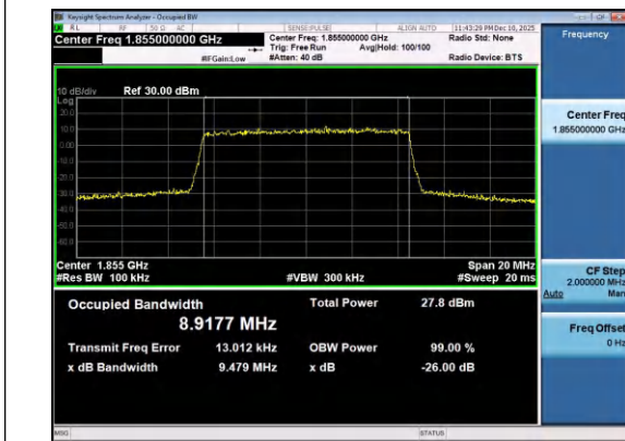
Band2-10MHz-QPSK-18650-50RB#0-PASS
