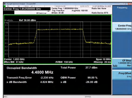
Band2-5MHz-QPSK-18625-25RB#0-PASS
