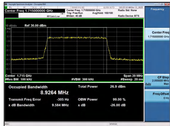
Band4-10MHz-QPSK-20000-50RB#0-PASS
