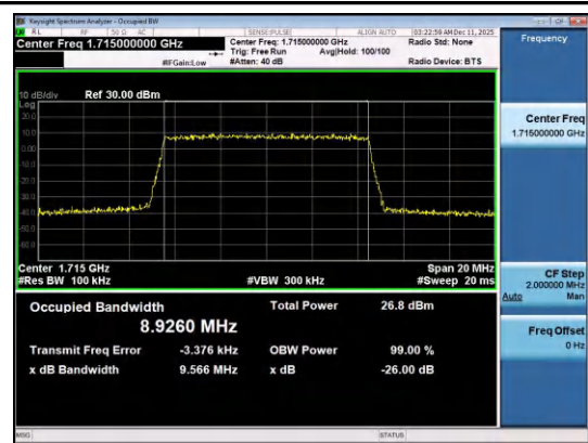
Band4-10MHz-QPSK-20000-50RB#0-PASS
