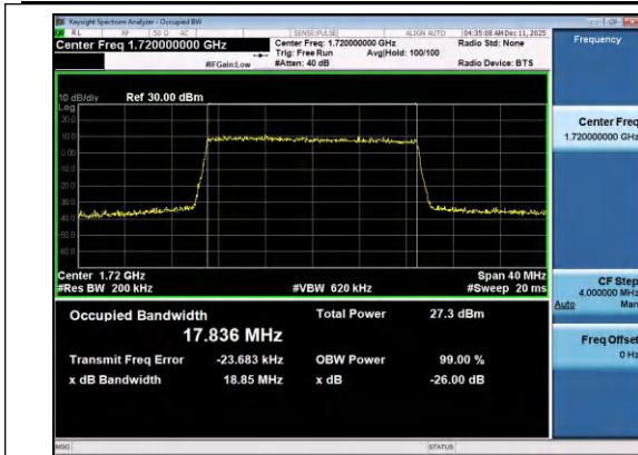
Band4-20MHz-QPSK-20050-100RB#0-PASS
