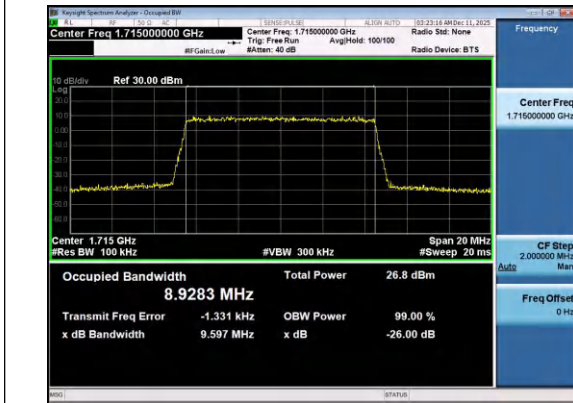
Band4-10MHz-QPSK-20000-50RB#0-PASS
