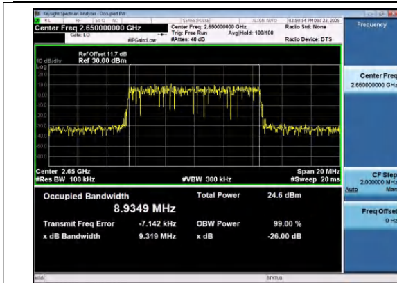
Band41(2535-2655)-10MHz-QPSK-41190-50RB#0-PA SS
