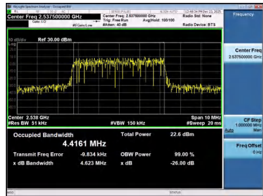
Band41(2535-2655)-5MHz-QPSK-40065-25RB#0-PAS
