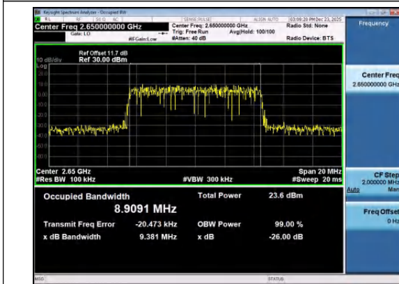
Band41(2535-2655)-10MHz-16QAM-41190-50RB#0-P ASS
