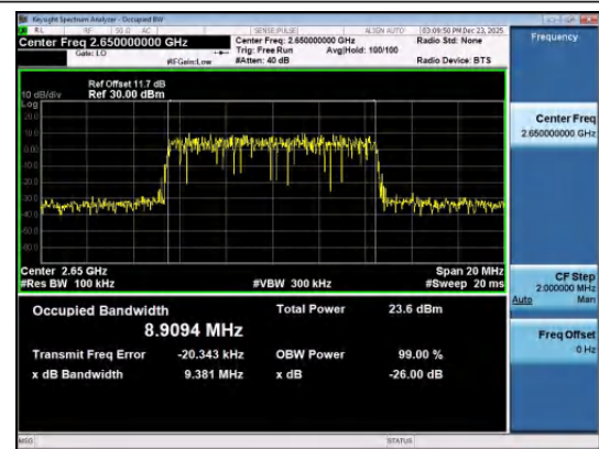
Band41(2535-2655)-10MHz-16QAM-41190-50RB#0-P ASS
