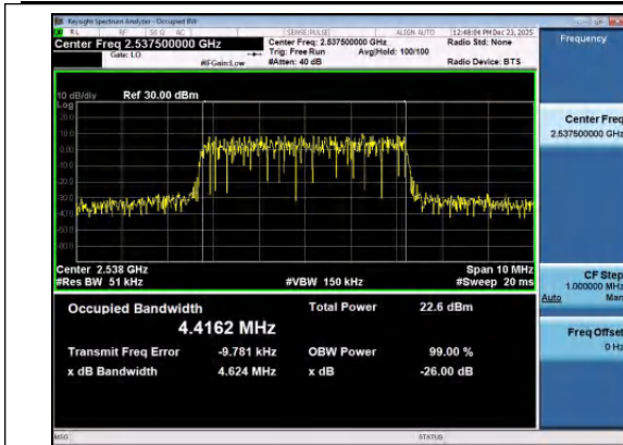
Band41(2535-2655)-5MHz-QPSK-40065-25RB#0-PAS
