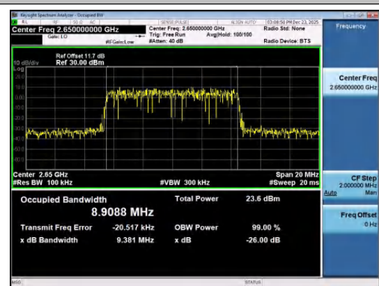
Band41(2535-2655)-10MHz-16QAM-41190-50RB#0-P ASS
