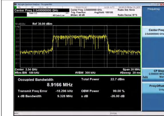
Band41(2535-2655)-10MHz-16QAM-40090-50RB#0-P ASS
