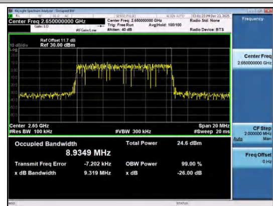
Band41(2535-2655)-10MHz-QPSK-41190-50RB#0-PA SS
