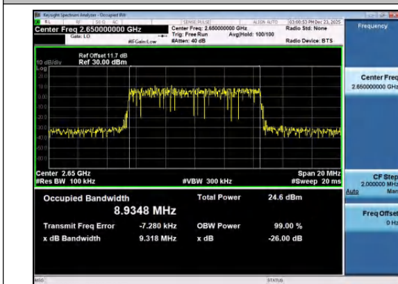
Band41(2535-2655)-10MHz-QPSK-41190-50RB#0-PA SS
