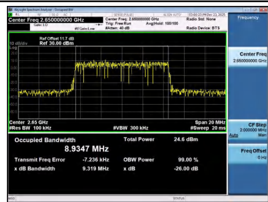
Band41(2535-2655)-10MHz-QPSK-41190-50RB#0-PA SS
