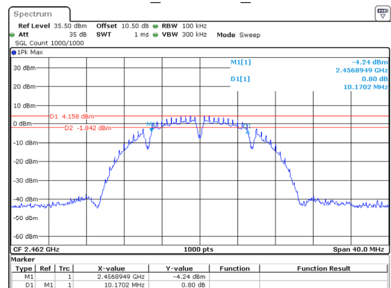
802.11b_2462MHz_Chain 1
