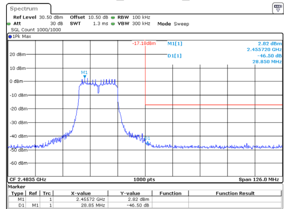
802.11n20_2462MHz_Chain 0
