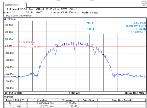
802.11b_2412MHz_Chain 1
