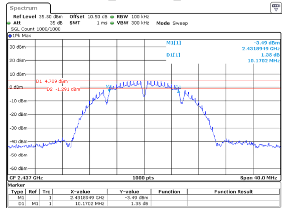
802.11b_2437MHz_Chain 0
