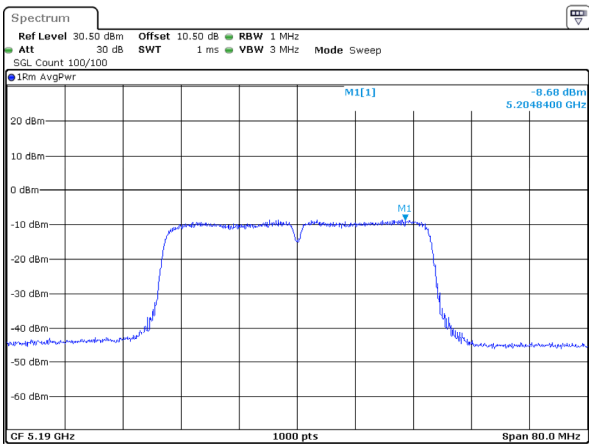
802.11ac40_5190MHz_Chain 0
