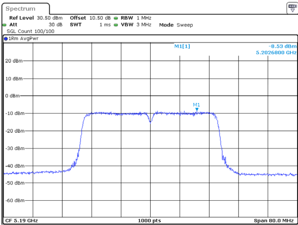
802.11ac40_5190MHz_Chain 1
