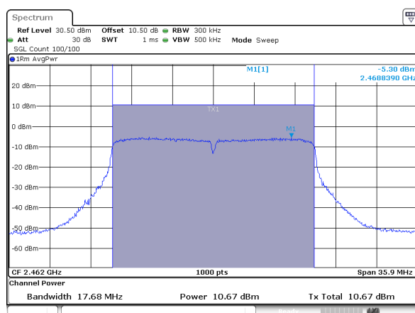
802.11n20_2462MHz_Chain 1
