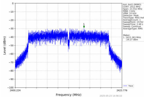
802.11n(HT20) LCH 2412MHz MIMO NTNv
