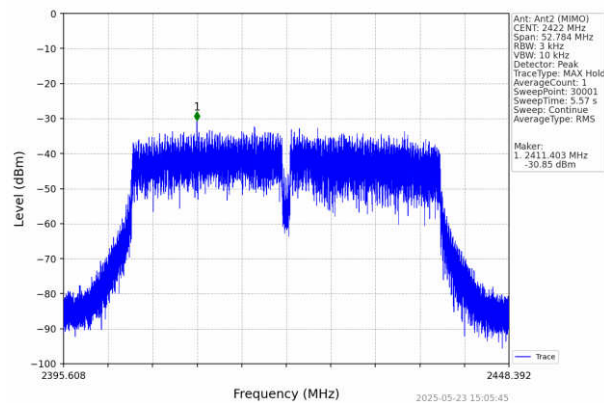
802.11n(HT40) LCH 2422MHz MIMO NTNv
