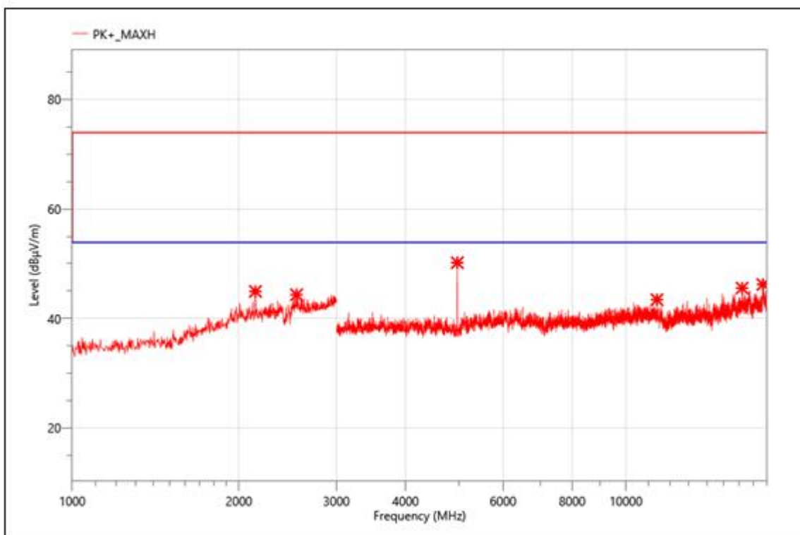
3-DH5 2480
