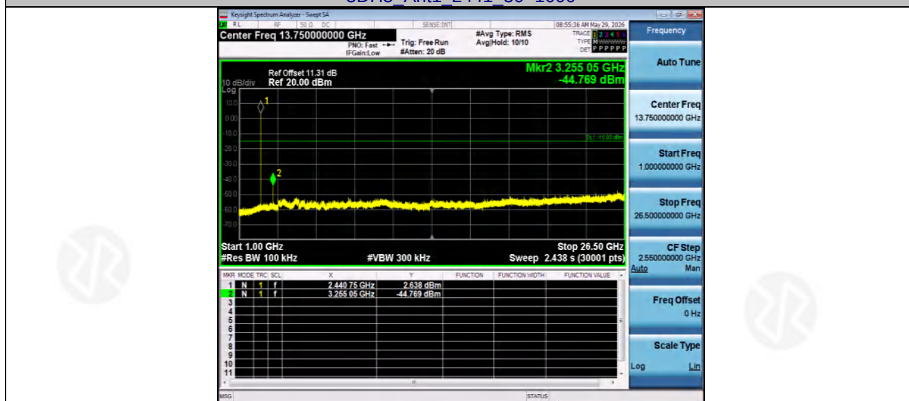
3DH5 Ant1 2441 1000~26500
