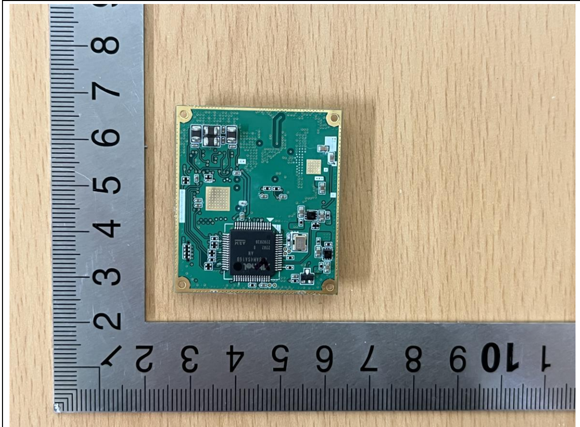
RFID Module
