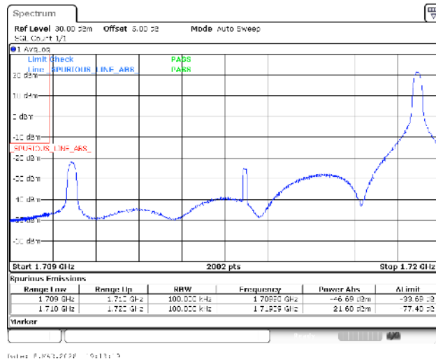
Band4-10MHz-QPSK-20000-1RB#49-PASS
