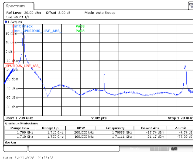
Band4-20MHz-QPSK-20050-1RB#0-PASS
