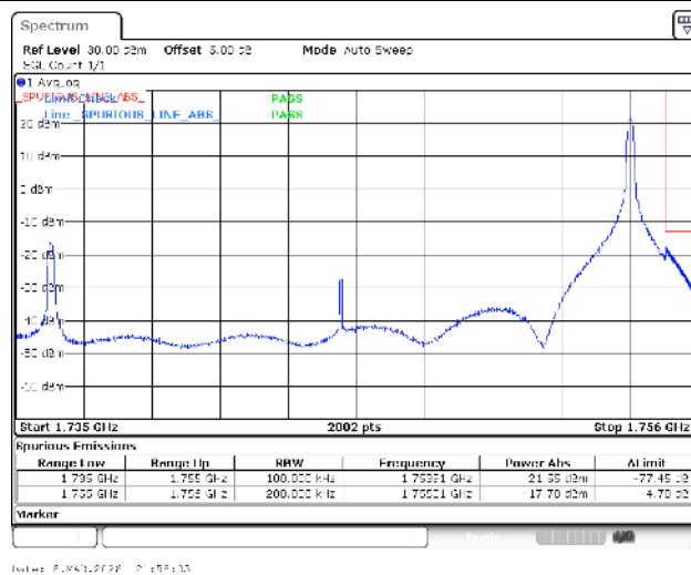
Band4-20MHz-QPSK-20300-1RB#99-PASS
