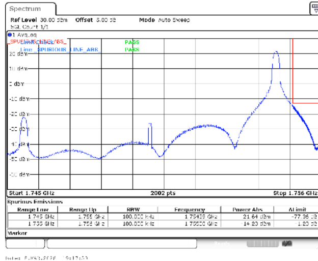
Band4-10MHz-QPSK-20350-1RB#49-PASS
