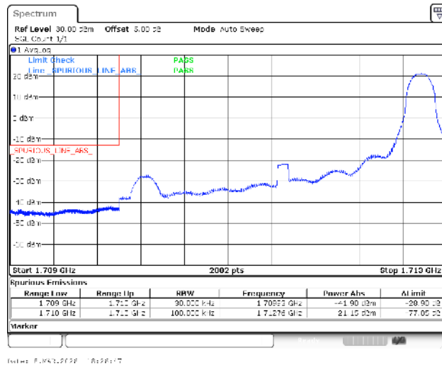
Band4-3MHz-QPSK-19965-1RB#14-PASS
